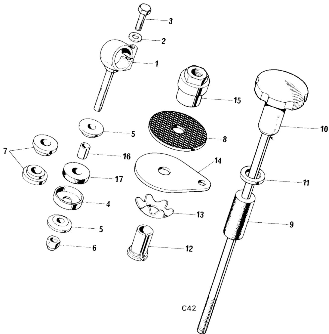
Fig. 30. STEERING DAMPER
