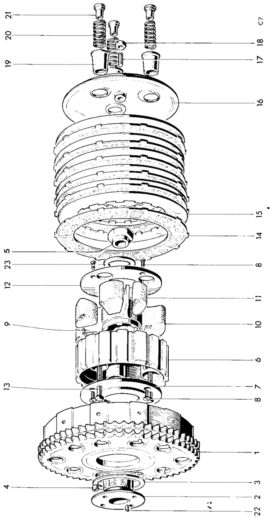
Fig. 13. CLUTCH
