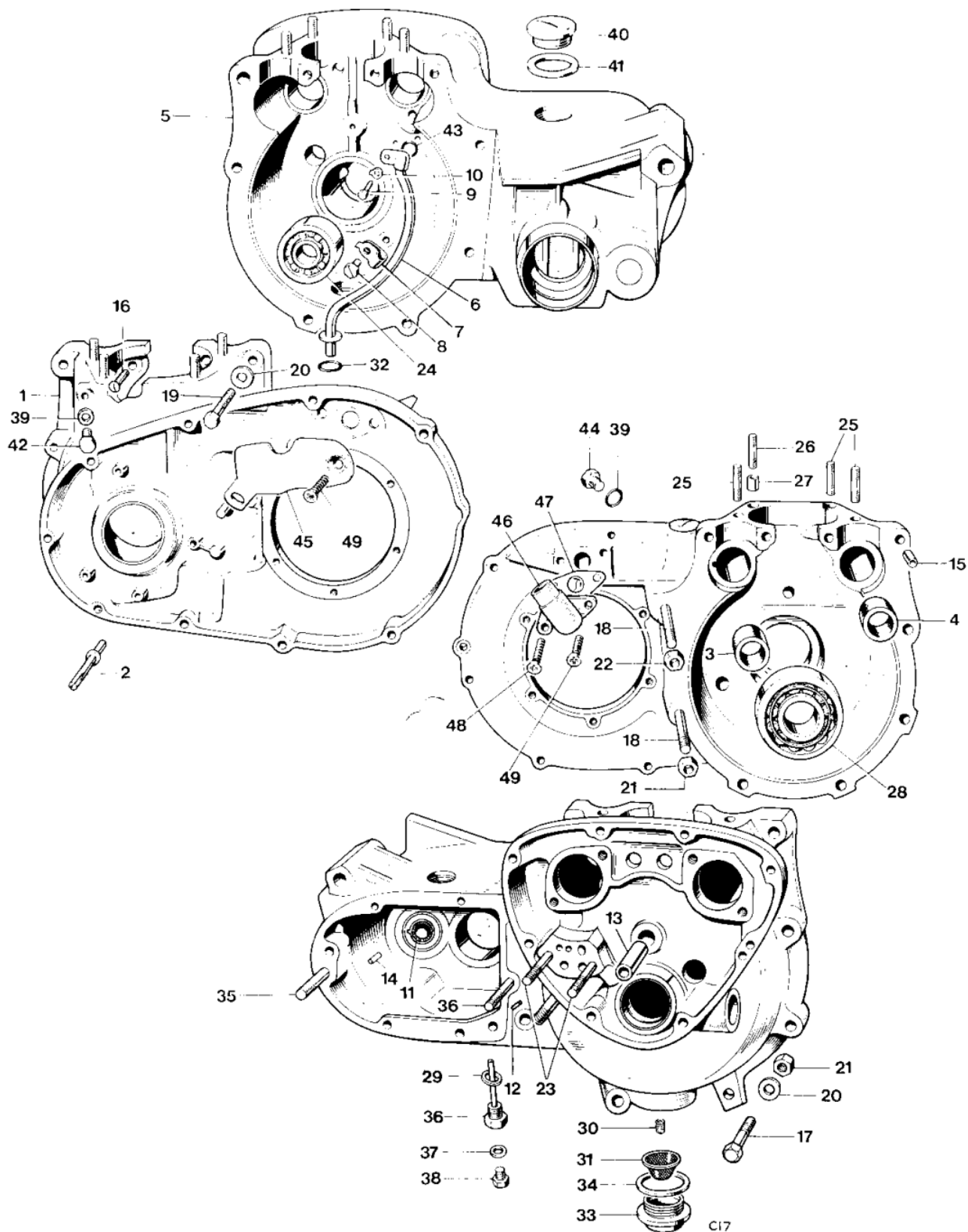
Fig. 2. CRANKCASE
