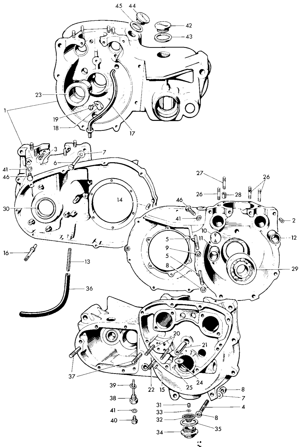
Fig. 2. CRANKCASE
