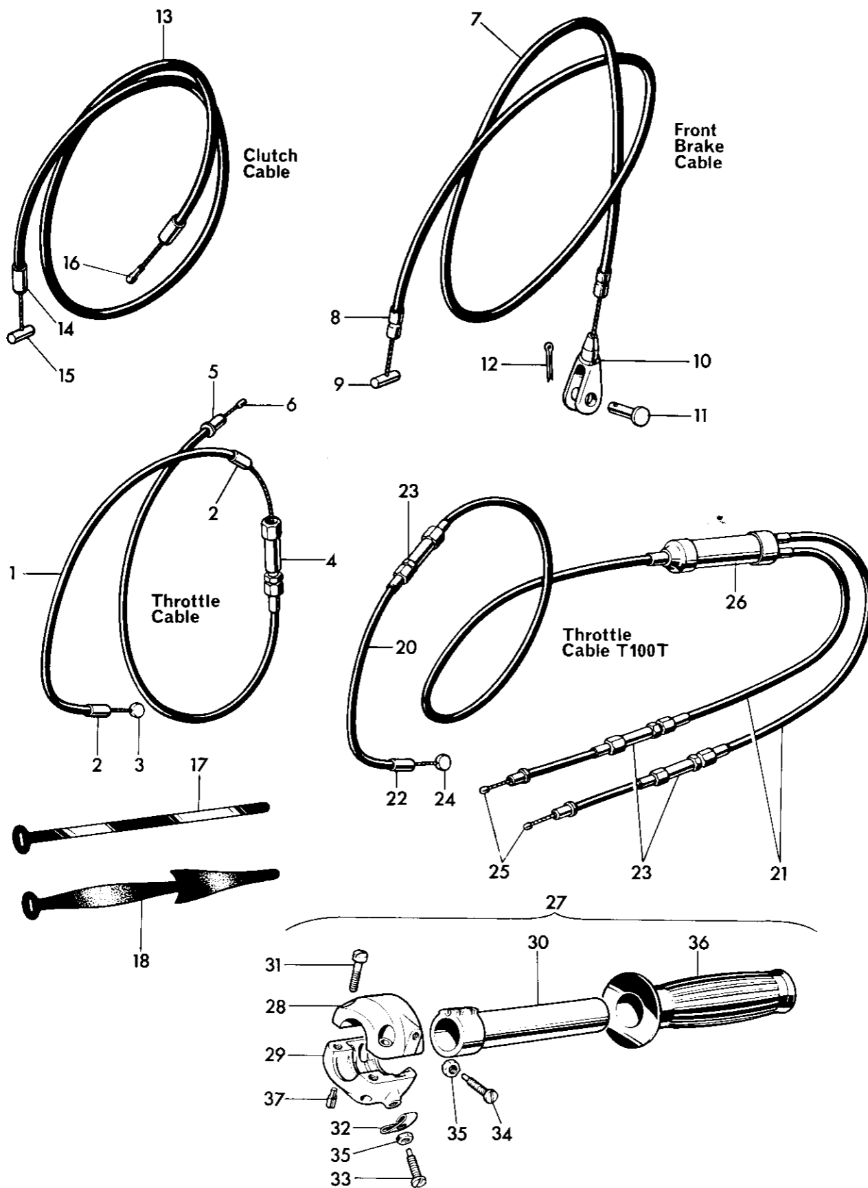
Fig. 28. CONTROL CABLES
