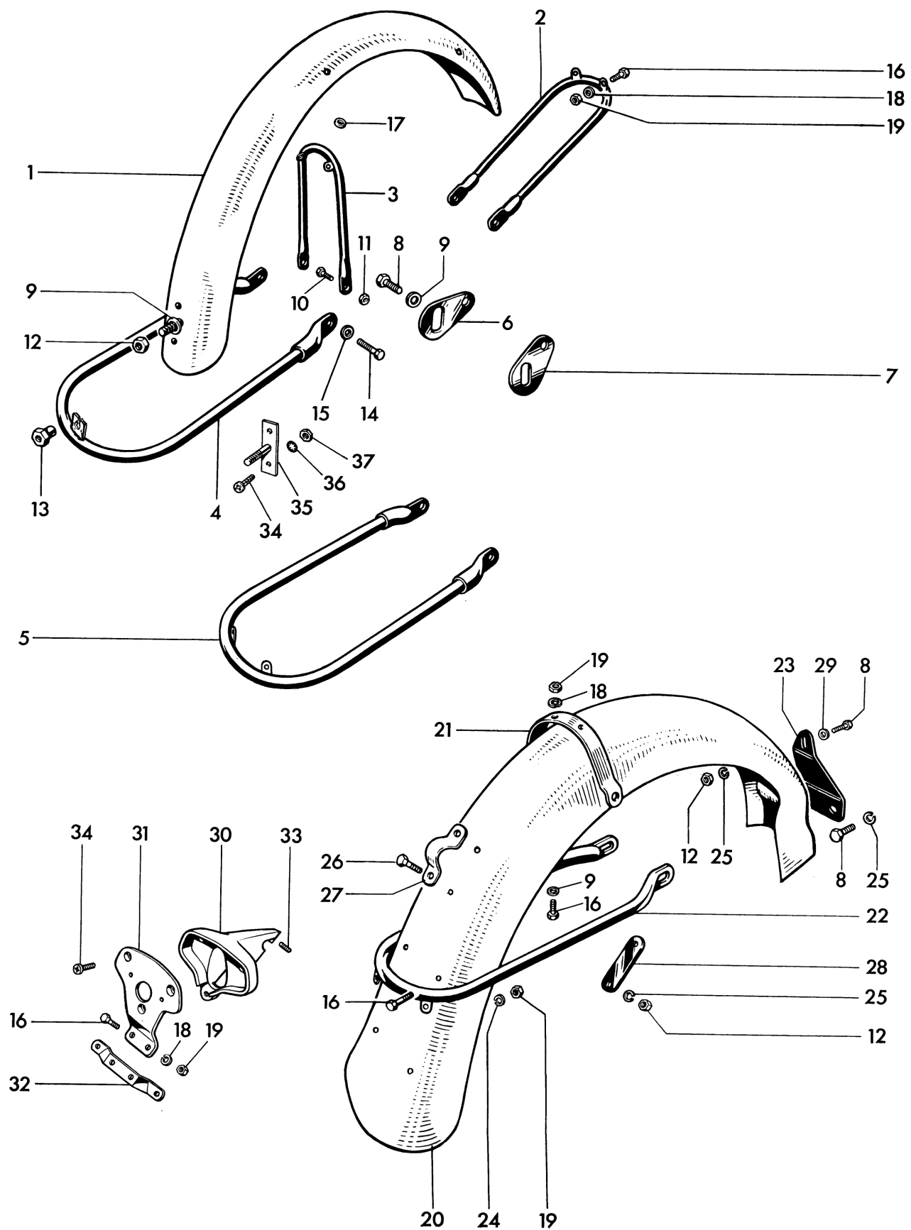
Fig. 30. FENDERS (U.S.A.)
