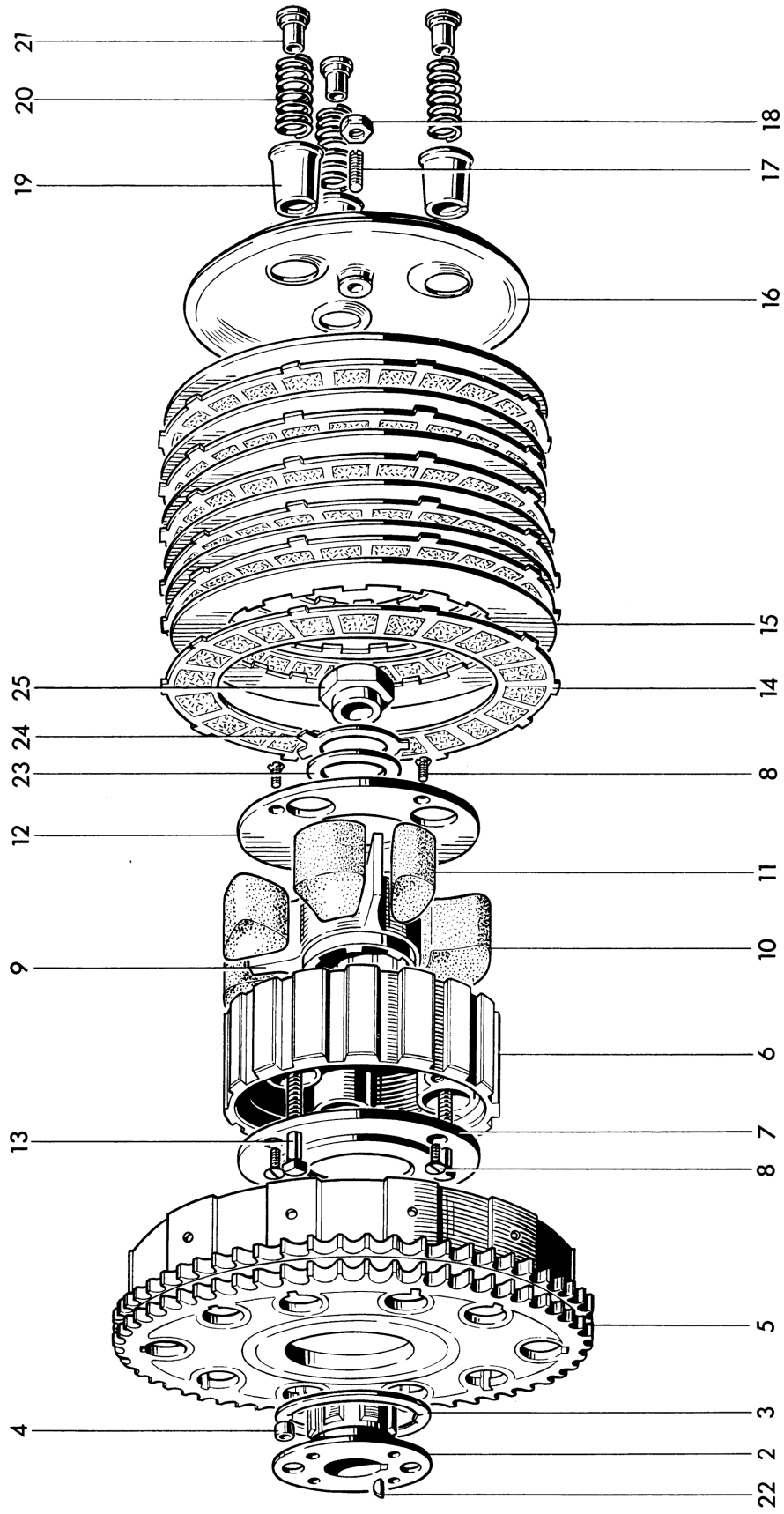
Fig. 10. CLUTCH
