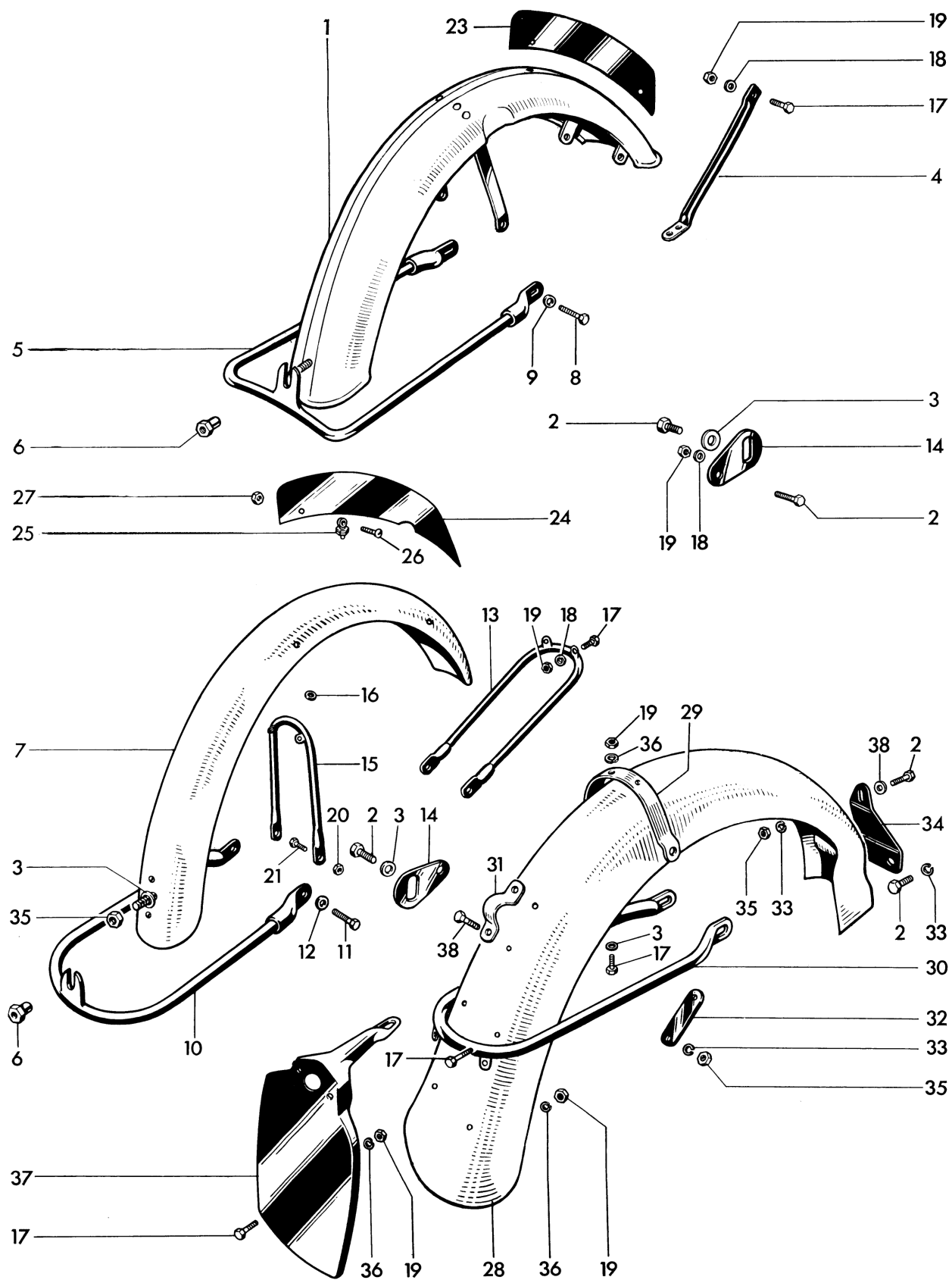
Fig. 29. MUDGUARDS (STANDARD)
