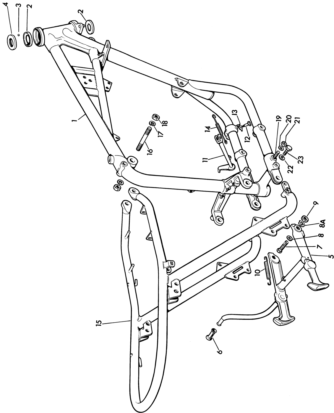
Fig. 12. FRAME
