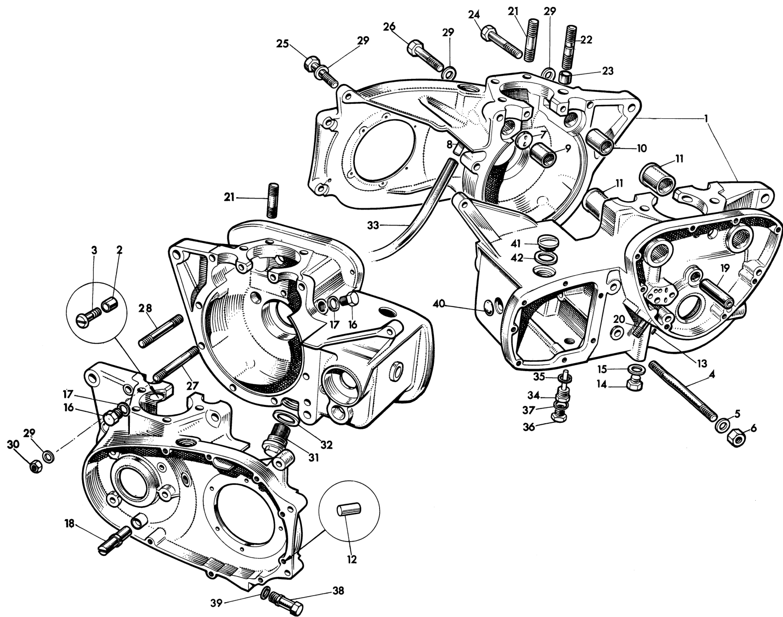
Fig. 2. CRANKCASE
