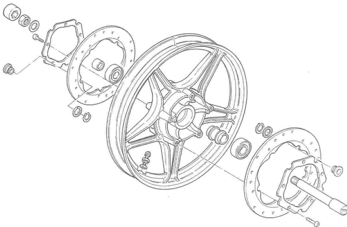
CERCHIO / RIM 18"x2.50" MT H2
