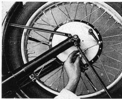
Bild 11. Vorderradbremse
