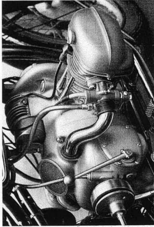
Bild 13. Motorblock R 51
