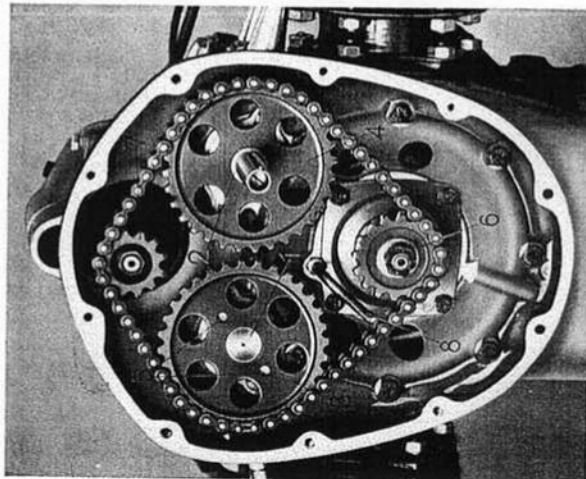
Bild 14. Stirnräderantrieb R 51
