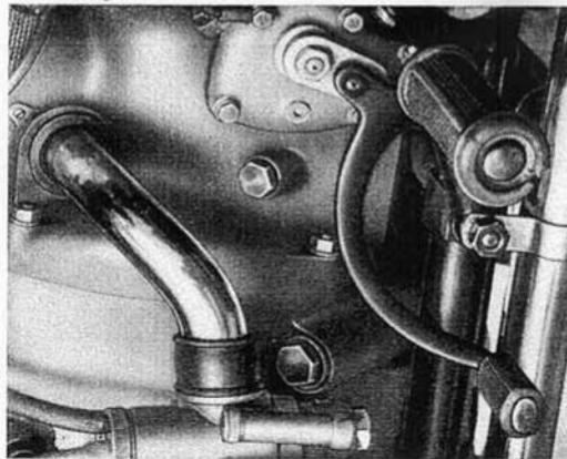
Bild 20. Fußschalthebel
