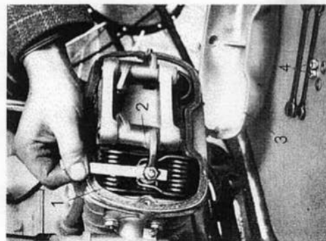
Bild 6. Zylinder-Kopf R 66 (R 55)
