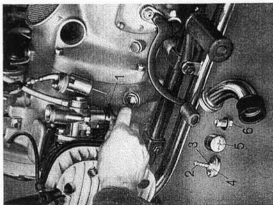
Bild 4. Vergaser R 71
