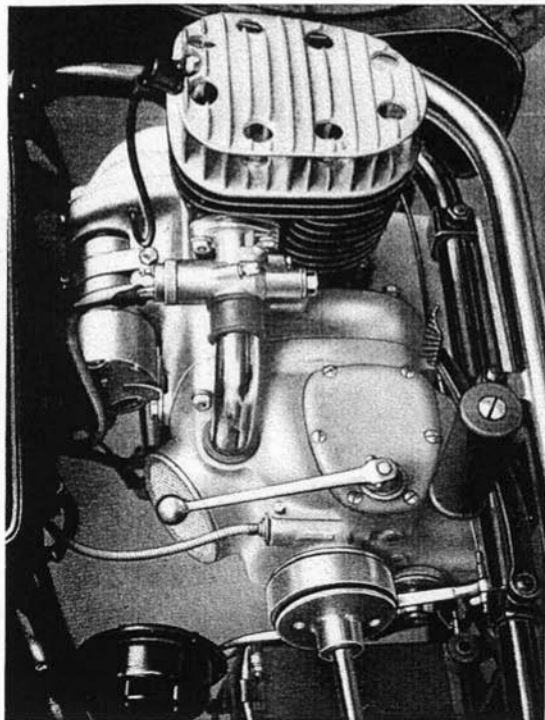
Bild 5. Motoranlage R 71
