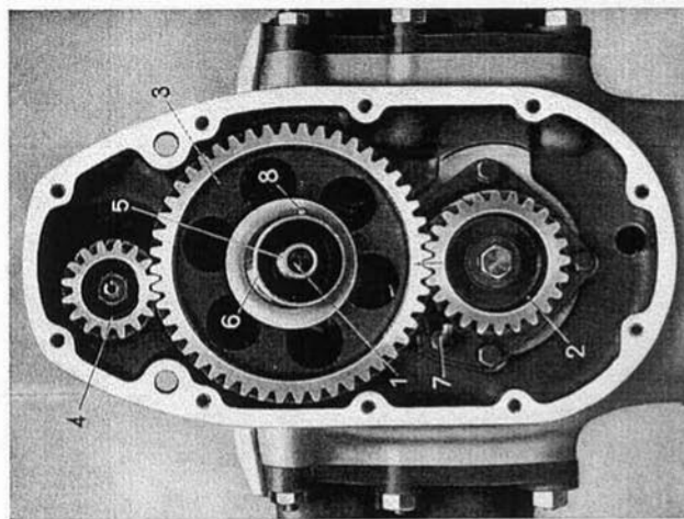
Bild 15. Stirnradantrieb R 61/66/71
