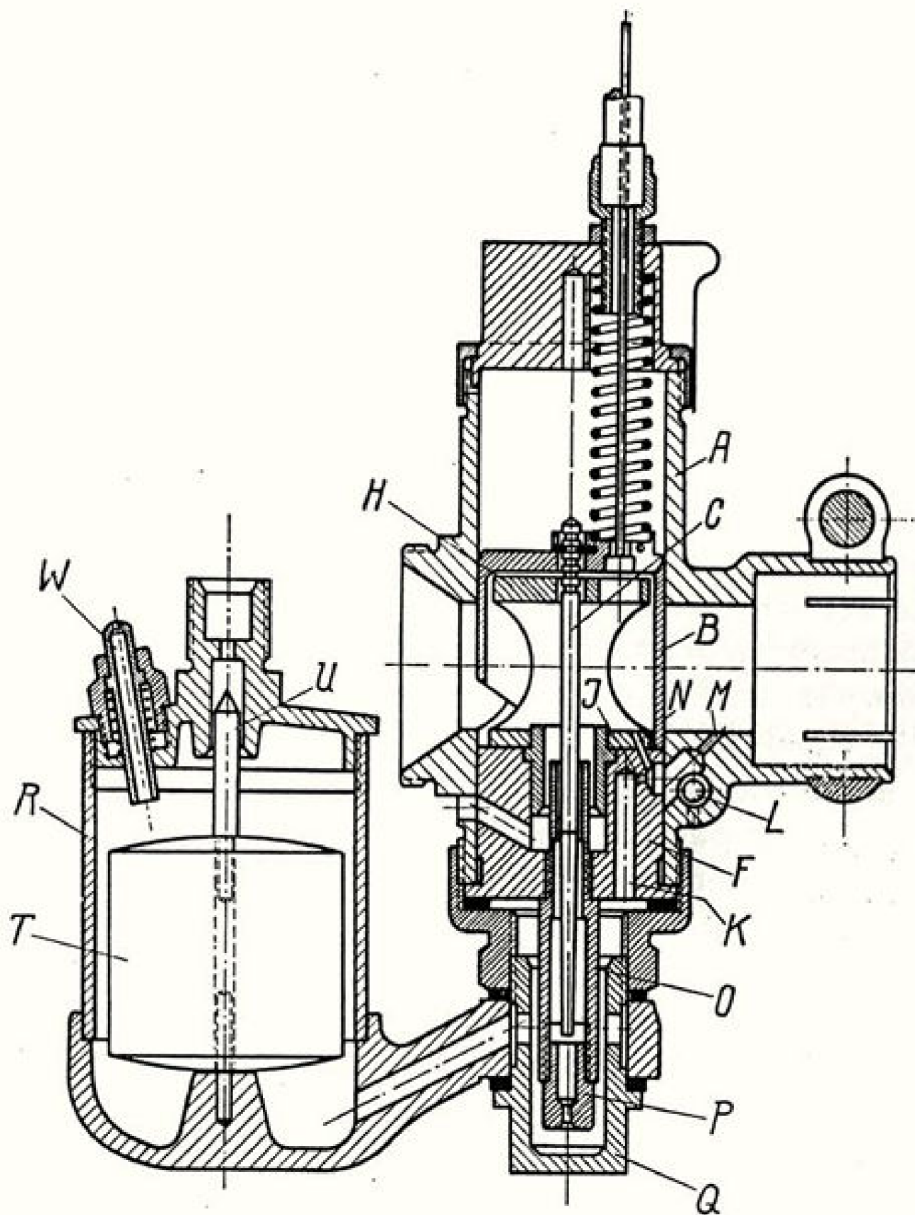
Abb. 25 Vergaser der Sportmaschine
