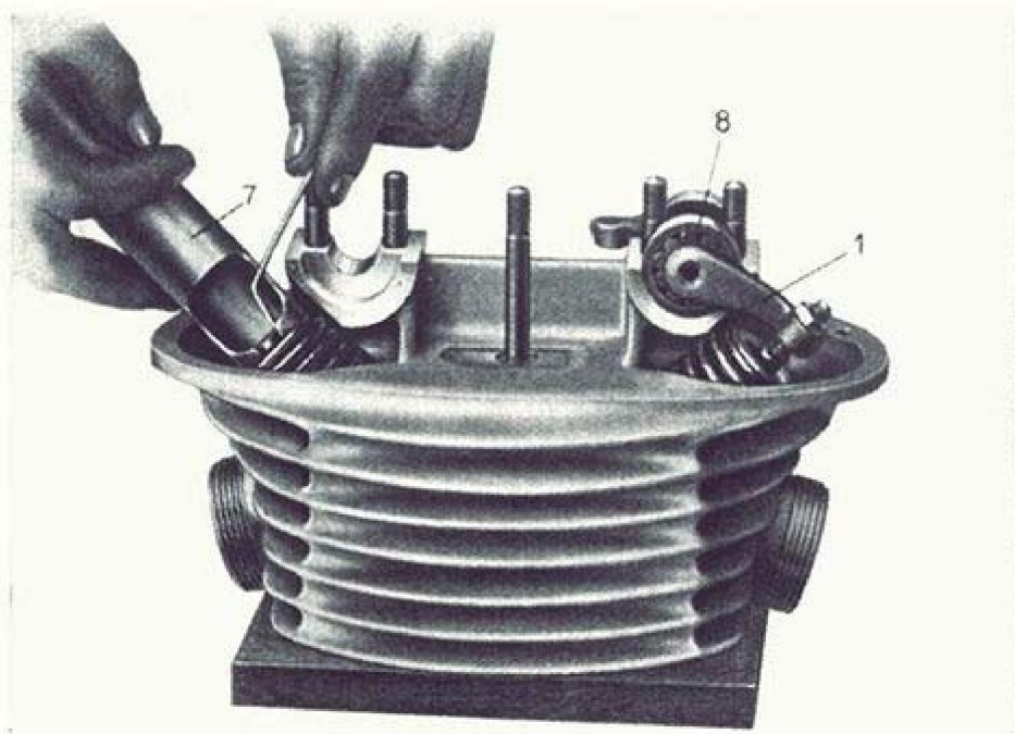
Abb. 35 Ausbau der Ventile bei der R 17-Maschine
