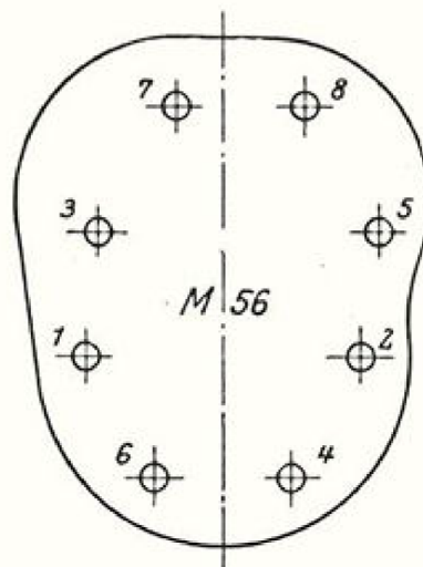
Abb. 9 Zylinderdeckel der Tourenmaschine
