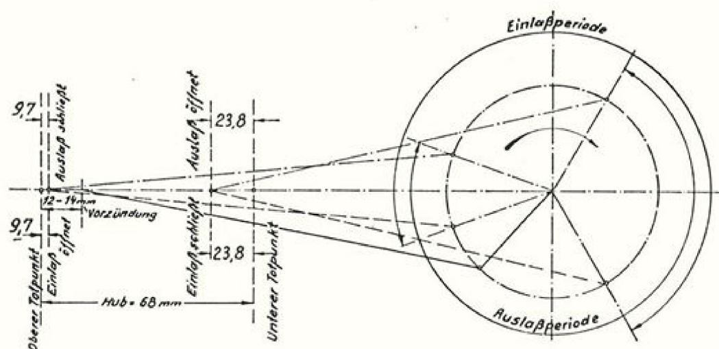
Abb. 38 Einstellschaubild für die Sportmaschine
