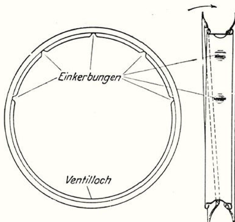
Abb. 42 Aufziehen von Drahtseilreifen auf Tiefbettsicherheitsfelgen
