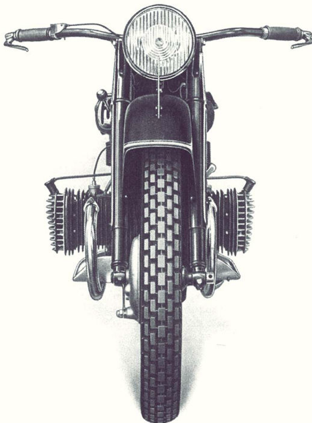
Abb. 31 Vorderansicht des R 12-Tourenrades
