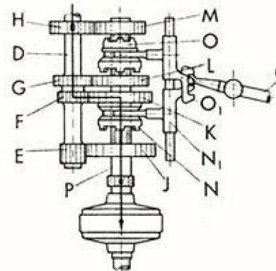
c) Kraftübertragung im 2. Gang
