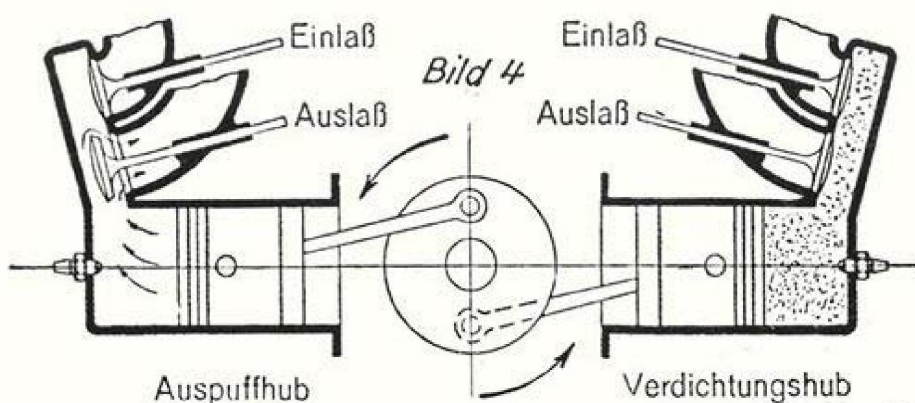
Abb. 19 Schaubildliche Darstellung der Arbeitsweise des Motors der R12-Tourenmaschine
