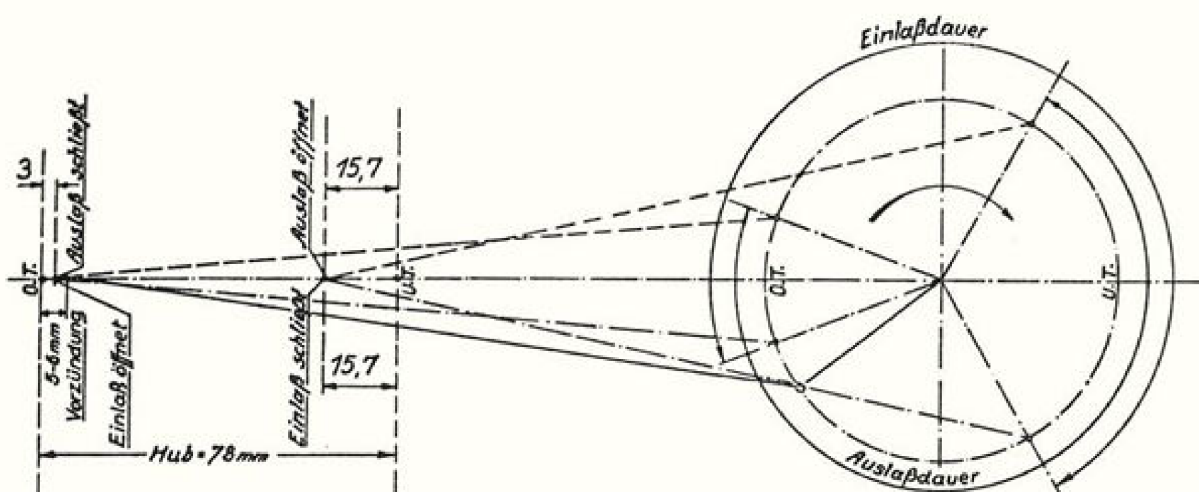
Abb. 37 Einstellschaubild für die Tourenmaschine
