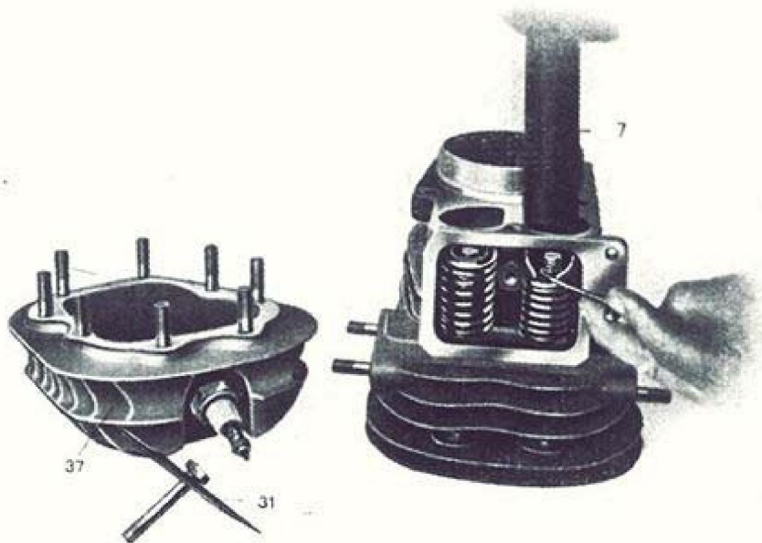
Abb. 34 Ausbau der Ventile bei der R 12-Maschine
