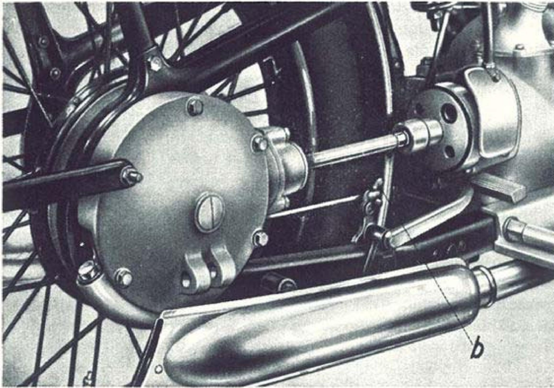
Abb. 11. Hinterradbremse
