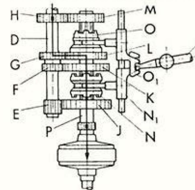
d) Kraftübertragung im 3. Gang
