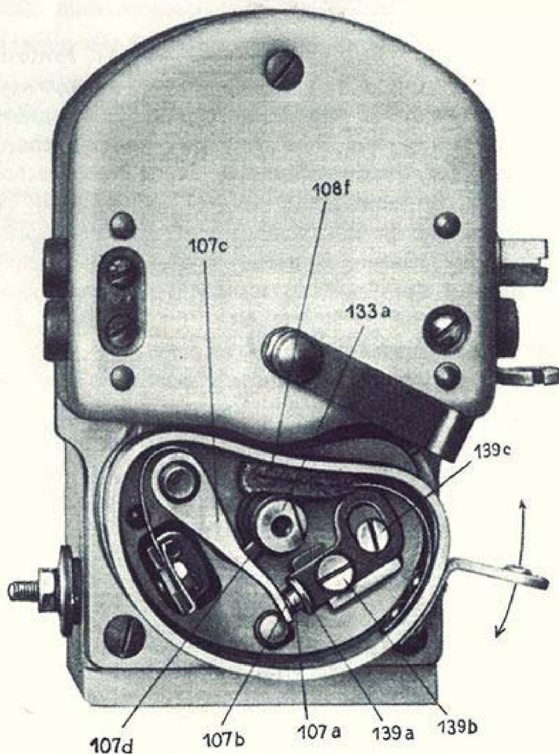
Abb. 12 Unterbrecher des Lichtbatteriezünders
