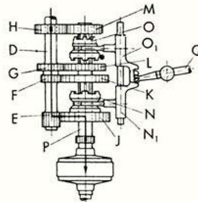
c) Kraftübertragung im 2. Gang
