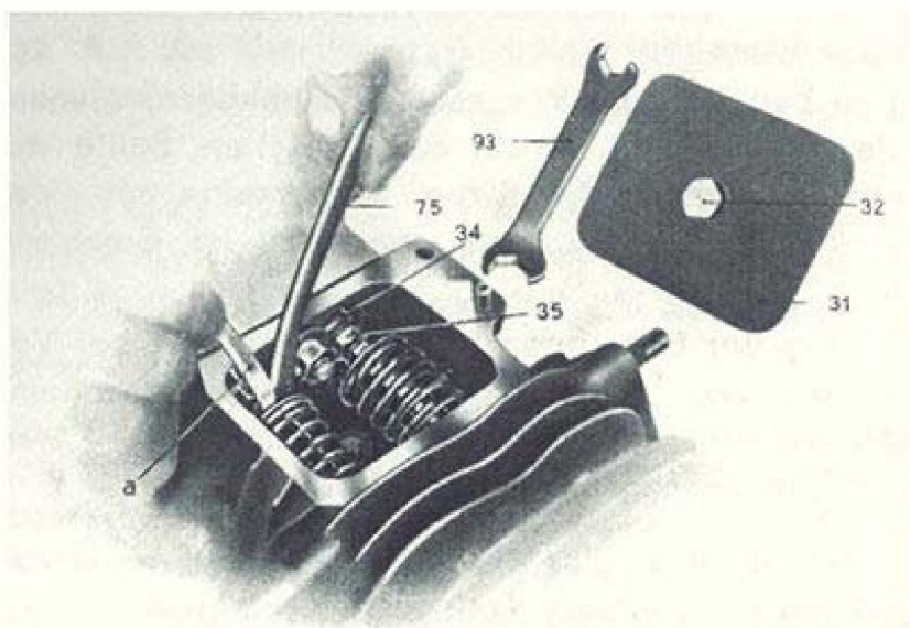
Abb. 14 Einstellen des Ventilspiels der Tourenmaschine
