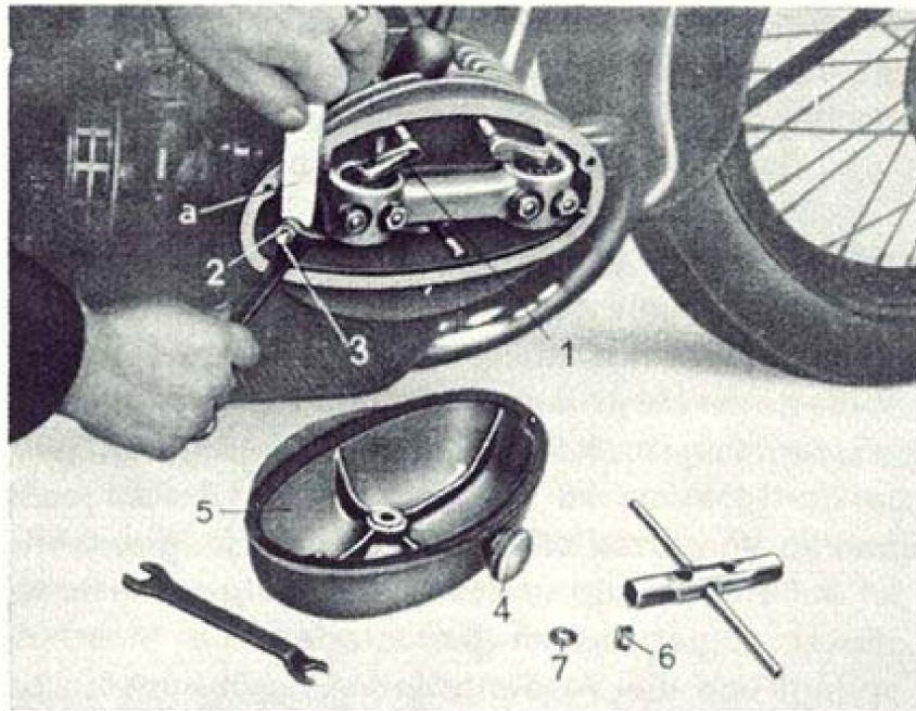
Abb. 15 Einstellen des Ventilspieles der Sportmaschine
