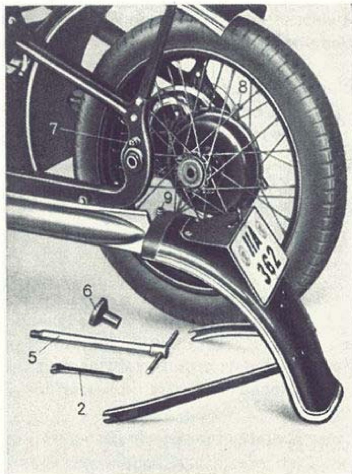
Abb. 41 Ausbau des Hinterrades bei Seitenwagenmaschinen
