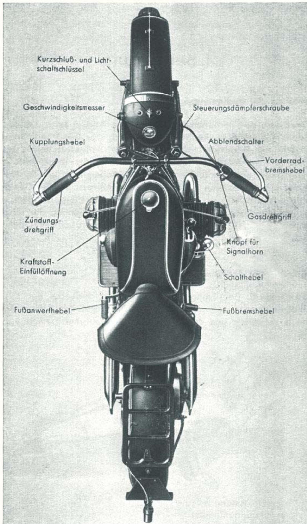
Abb. 6 Die Bedienungshebel am BMW-Kraftrad
