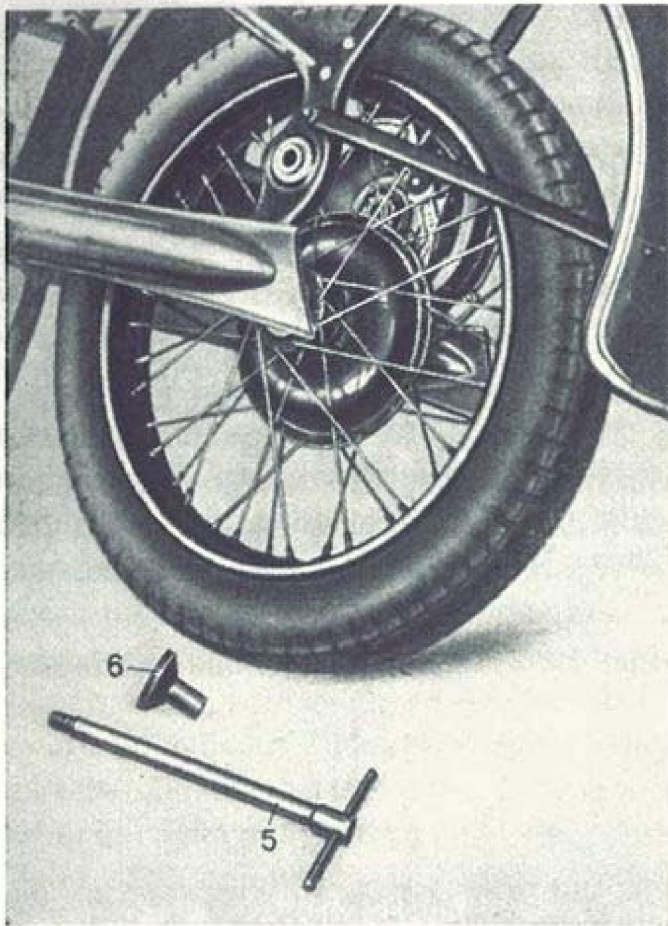
Abb. 40 Ausbau des Hinterrades bei Einzelmaschinen
