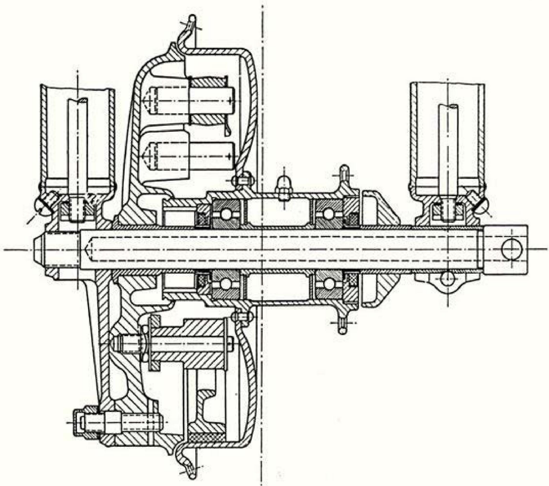
Abb. 32 Schnitt durch die Vorderradnabe und -bremse
