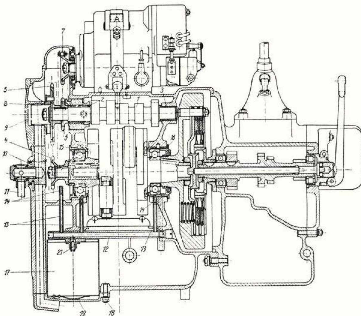
Abb. 22 Längsschnitt durch Motor und Getriebe
