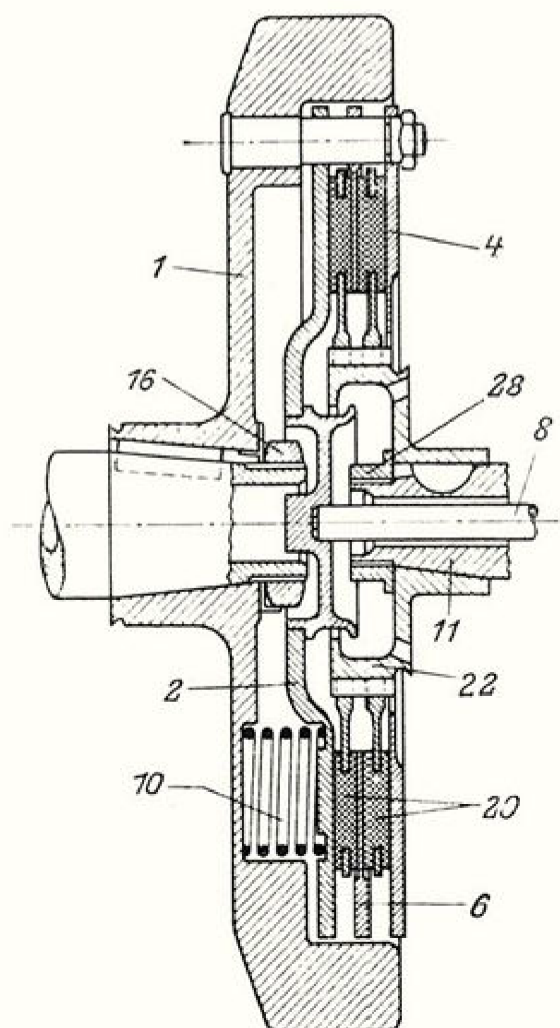
Abb. 26 Zweischeiben- Reibungskupplung
