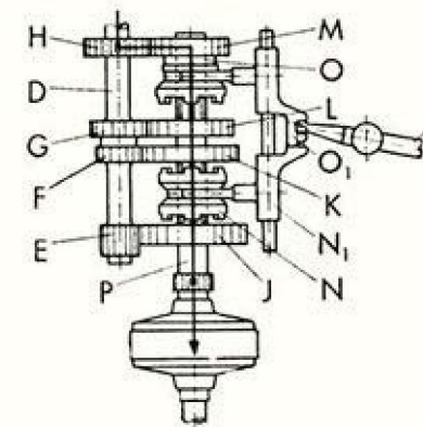
Abb. 27 Schema des Antriebes
