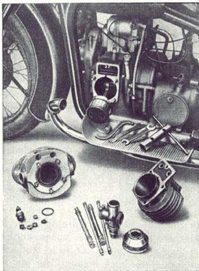
Abb. 21 Motor und Getriebe der R 17-Maschine mit abgenommenem Zylinder
