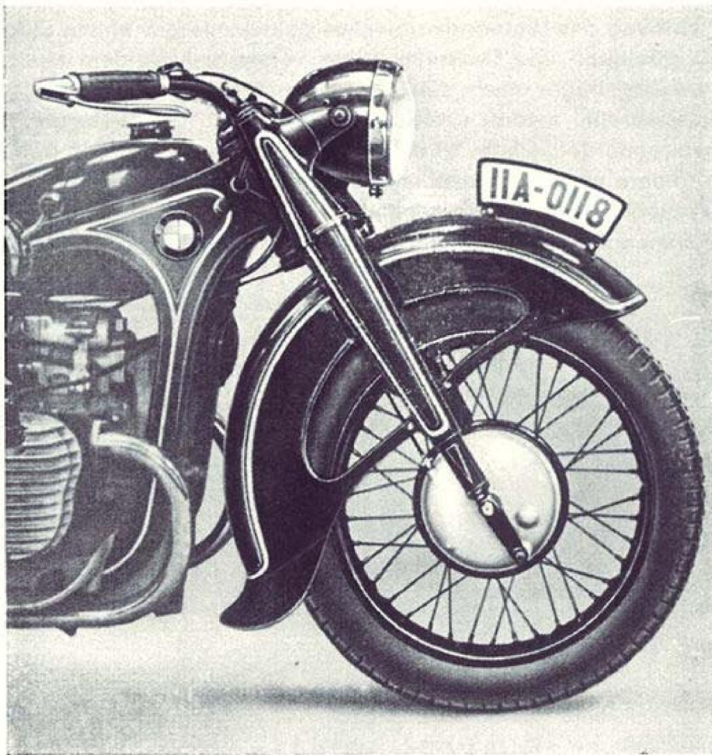
Abb. 30 Vorderrad mit Gabel und Scheinwerfer
