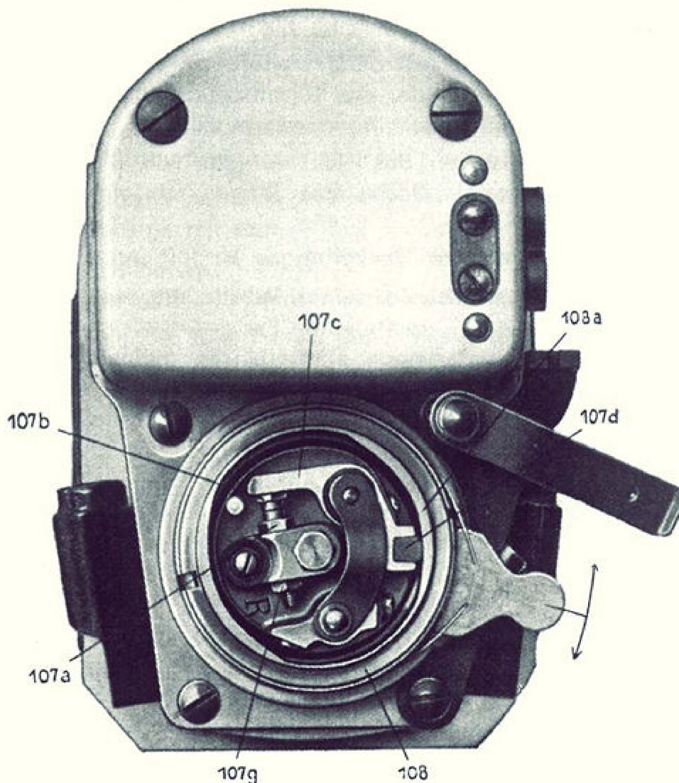
Abb. 13 Unterbrecher des Lichtmagnetzünders
