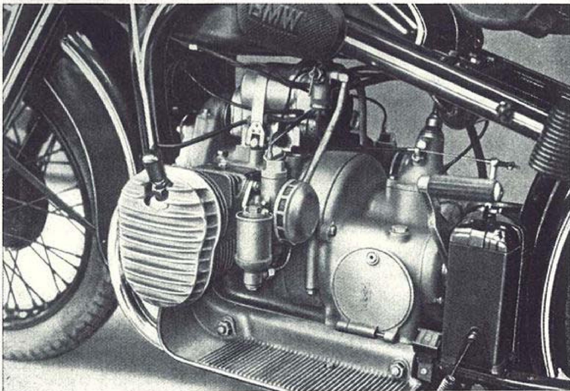
Abb. 16 Motor und Getriebe der R 12-Zweivergaser-Maschine
