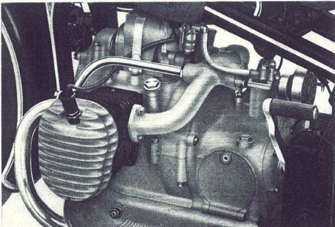
Abb. 18 Motor und Getriebe der R 12-Einvergaser-Maschine
