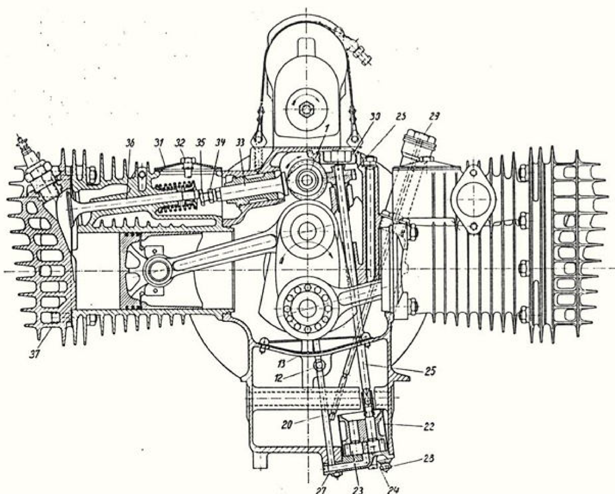
Abb. 36 Tourenmotor mit teilweisem Querschnitt durch die Zylindermitte
