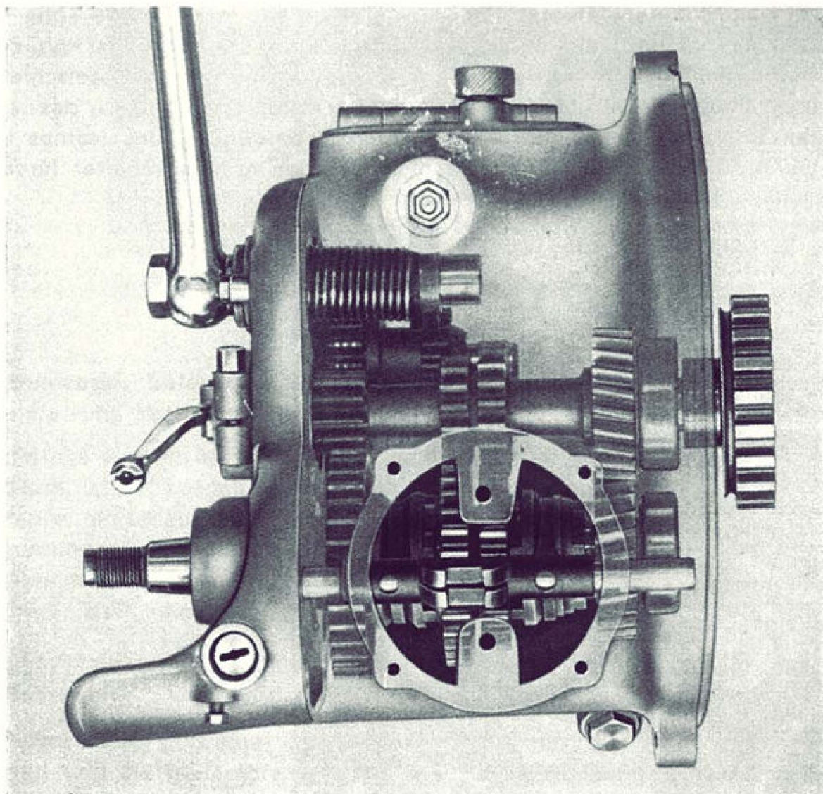
Abb. 28. Getriebe der Baumuster R 12 und R 17.
