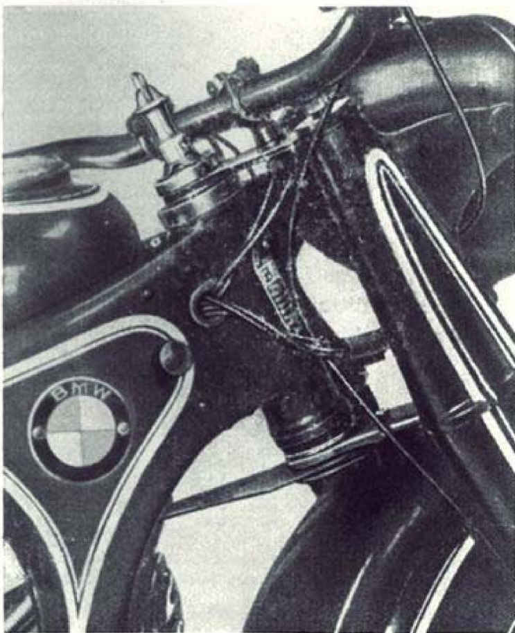
Abb. 29 Steuerkopf und Steuerungsdämpfer
