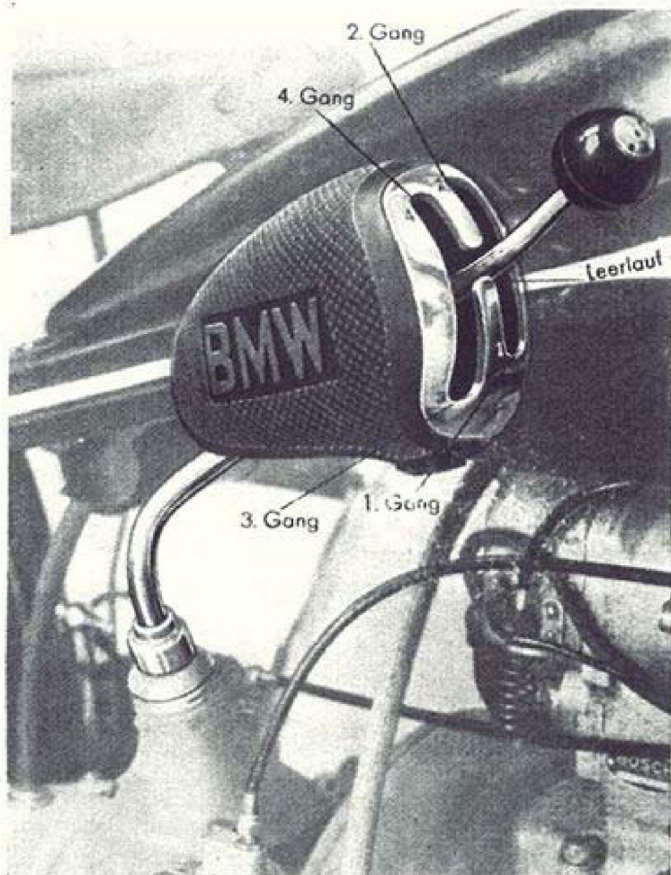
Abb. 8 Getriebebeschaltethebel
