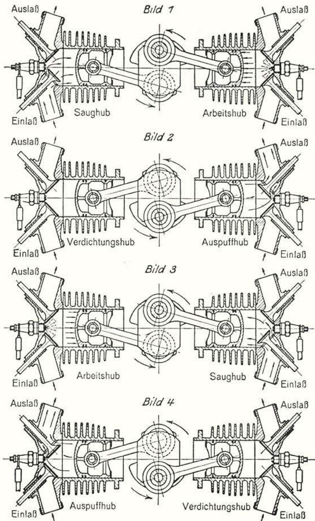
Abb. 20 Schaubildliche Darstellung der Arbeitsweise des Motors der R 17-Sportmaschine
