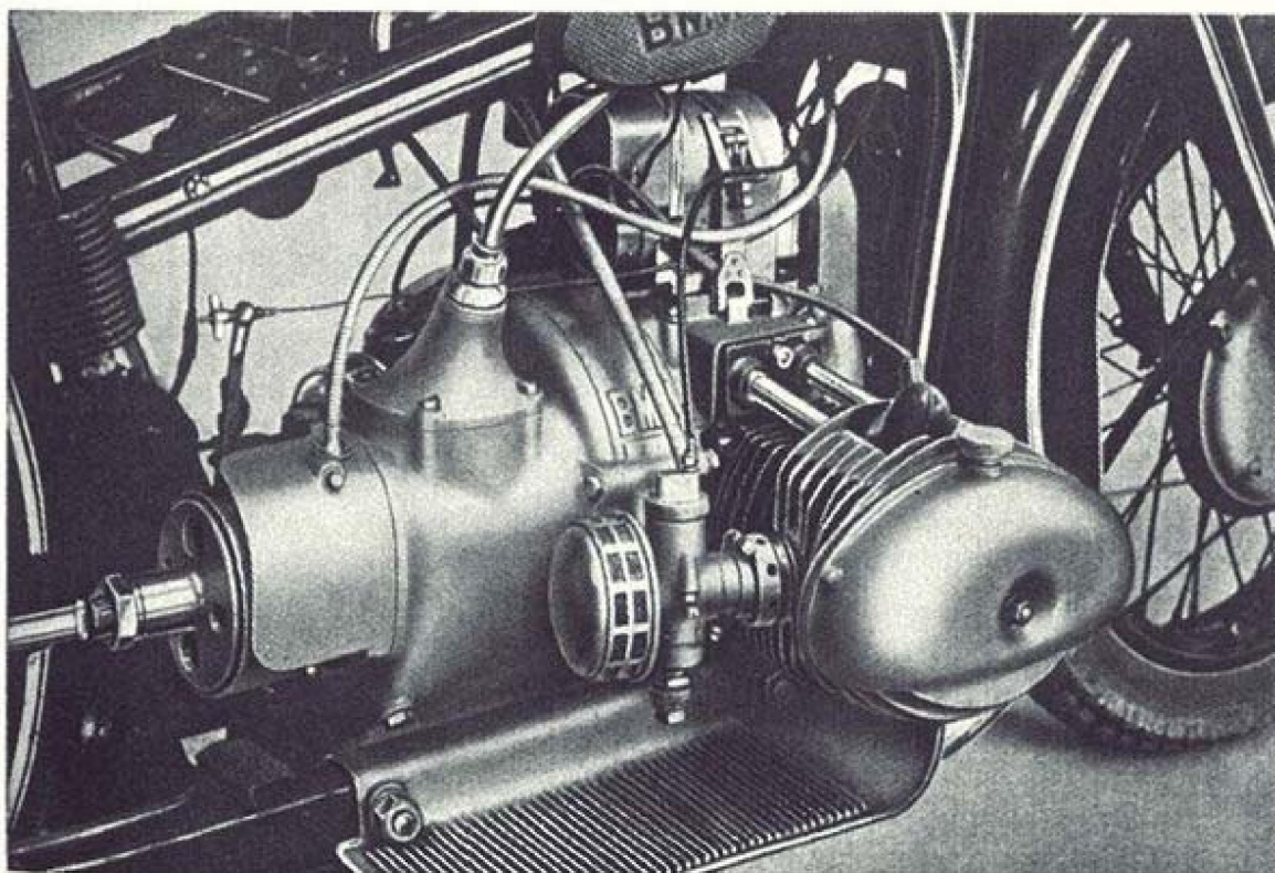
Abb. 17 Motor und Getriebe des R 17-Sportrades
