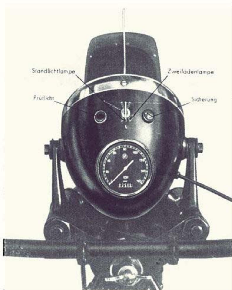
Abb. 33 Scheinwerfer von oben mit Stellungen des Schaltschlüssels
