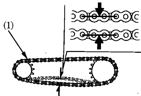
(1) Cadena de transmisión
