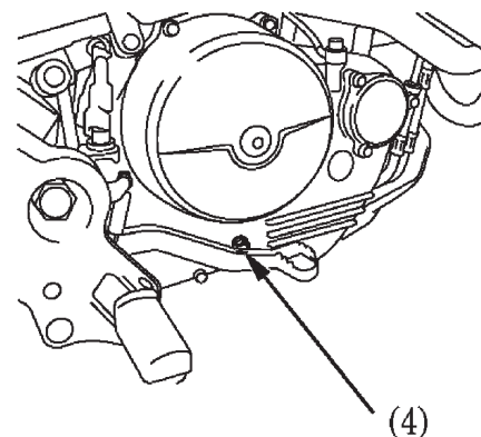
(4) Tornillo de comprobación del nivel de aceite del cárter
