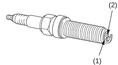
(1) aislador de porcelana (2) electrodo central
