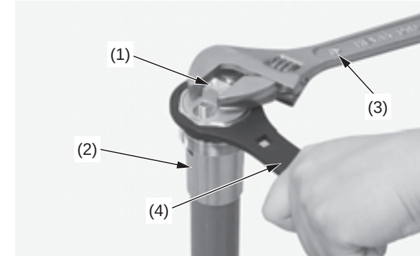
(1) conjunto de la tapa de la horquilla (2) amortiguador de la horquilla (3) llave ajustable (4) llave de contratuercas
