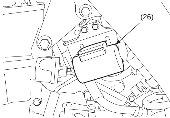
(26) condensador
