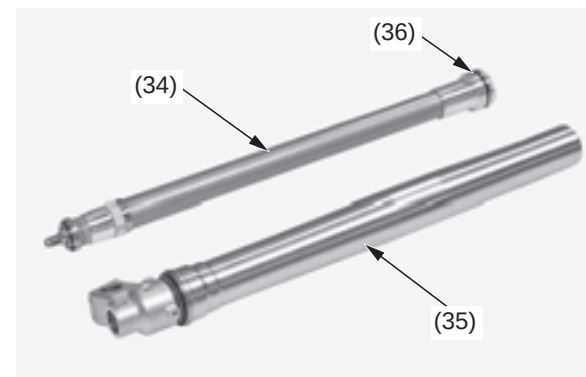
(34) conjunto del amortiguador de la horquilla (35) conjunto de la horquilla (36) junta tórica
