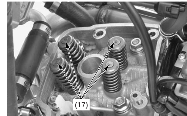
(17) laminillas
