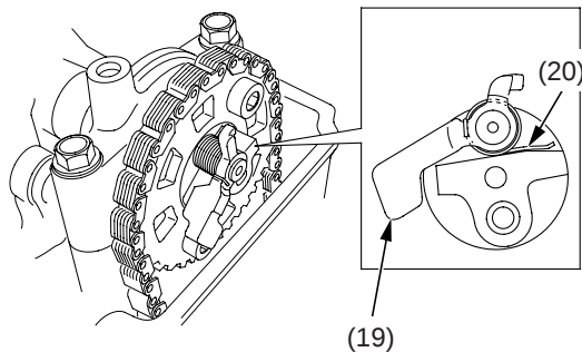
(19) contrapeso del descompresor (20) resorte de retorno
