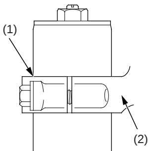
(1) ranura (2) abrazadera de la horquilla superior
