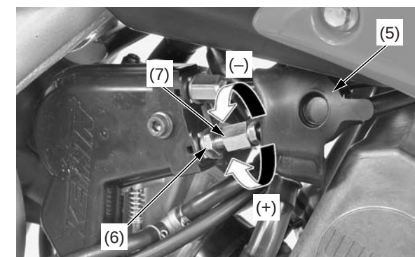
(5) cubierteira contra el polvo (6) contratuerca (7) ajustador (+) incrementar (-) reducir
