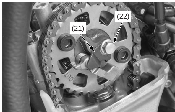
(21) placa de tope (22) perno
