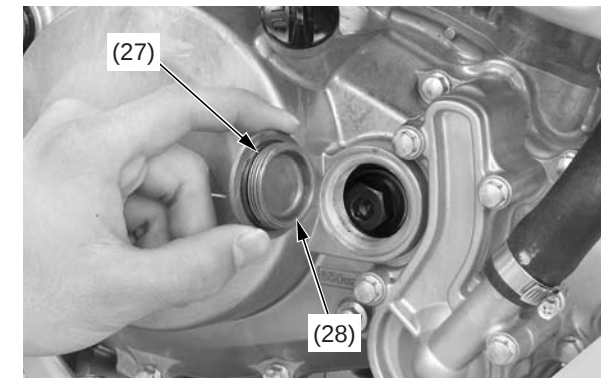
(27) junta tórica (28) tapa del orificio del cigüeñal
