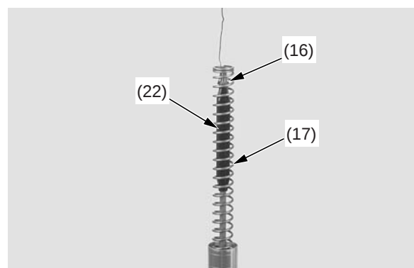
(16) contratuerca
