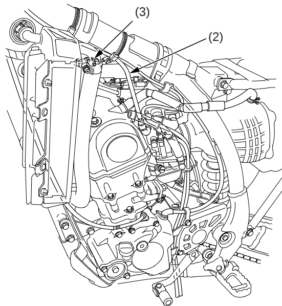
(1) cables del acelerador (2) cable de arranque en caliente (3) conector del sensor del acelerador
