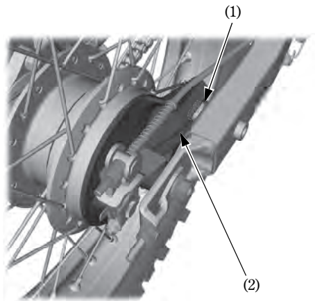
(1) Lug
