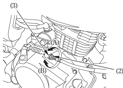
(2) Contratuerca (A) Aumenta el juego libre (3) Tuerca de ajuste (B) Disminuye el juego libre
