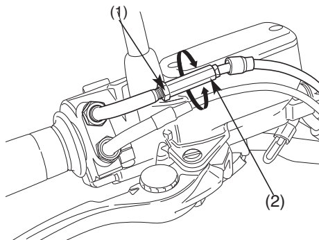
(1) Contratuerca
