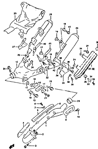
FIG.13 MUFFLER (C-5)
