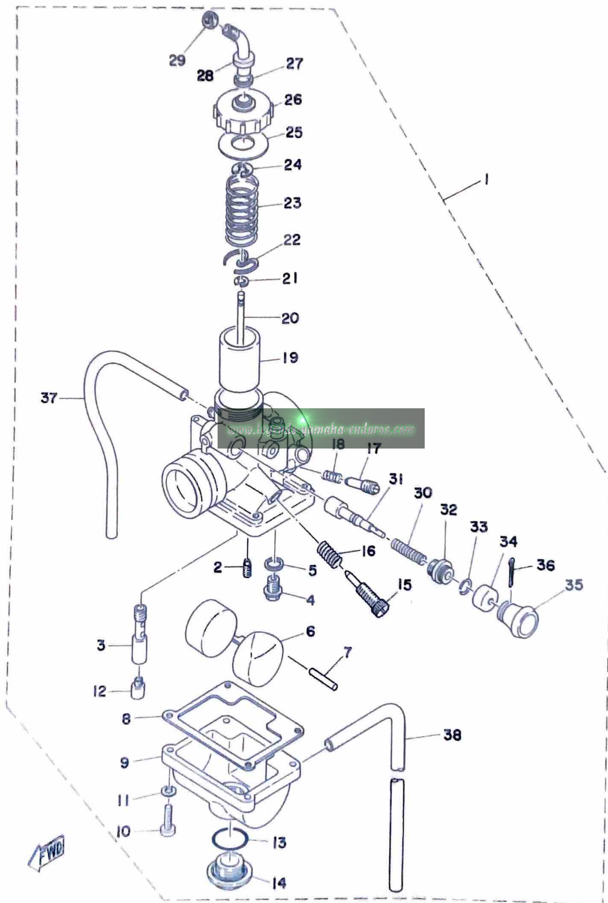
Fig. 10 CARBURETOR
