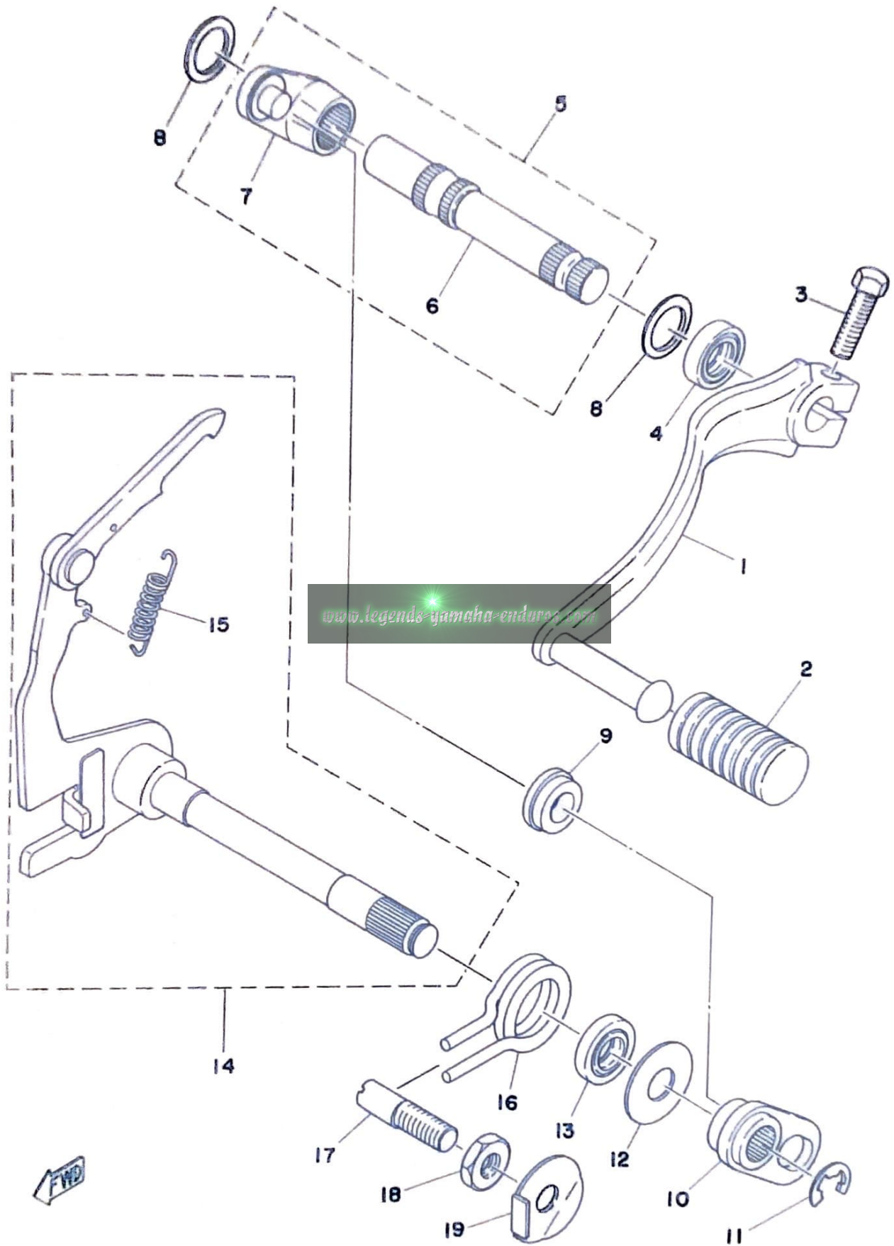
Fig. 7 SHIFTER 2
