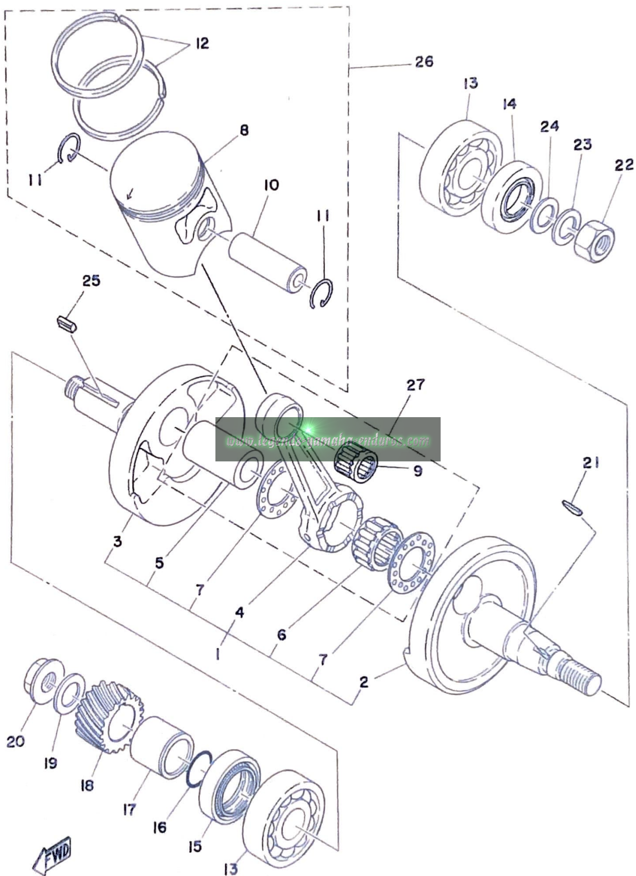
Fig. 3 CRANK · PISTON
