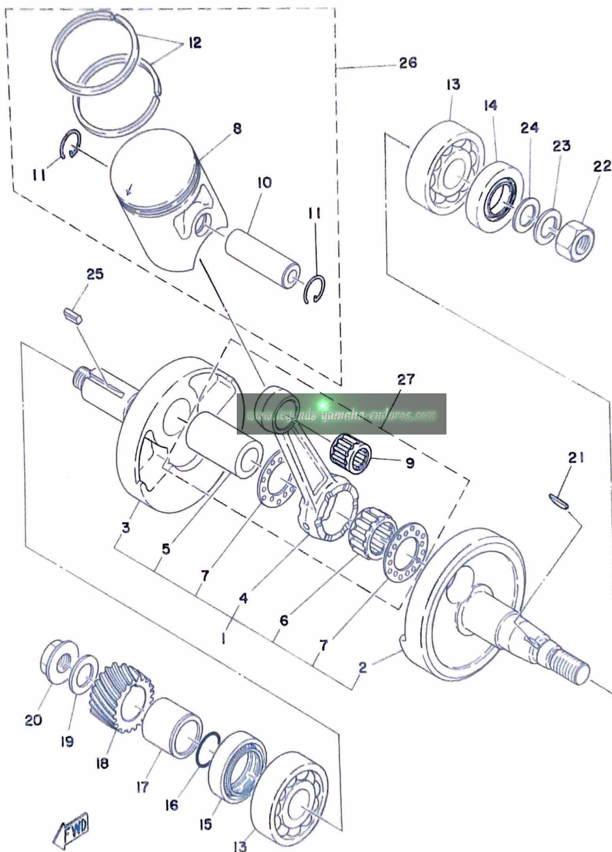
Fig. 3 CRANK · PISTON
