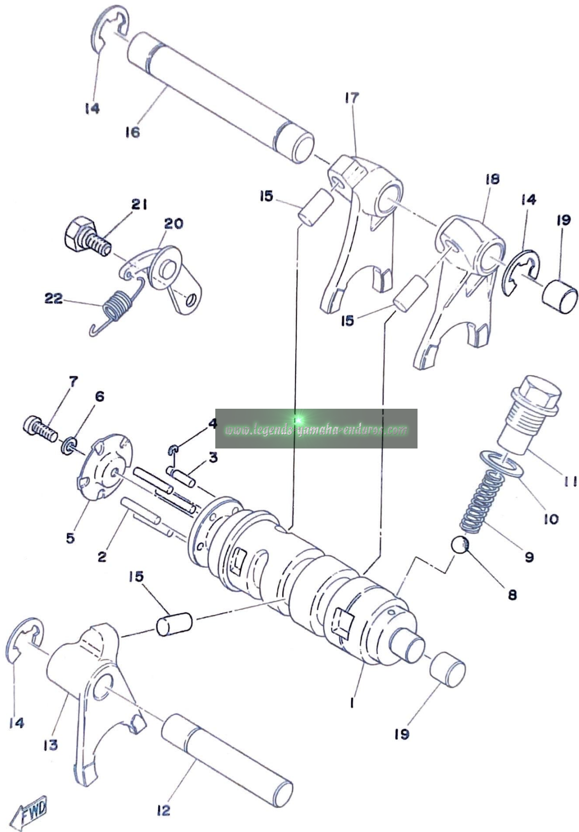
Fig. 6 SHIFTER 1
