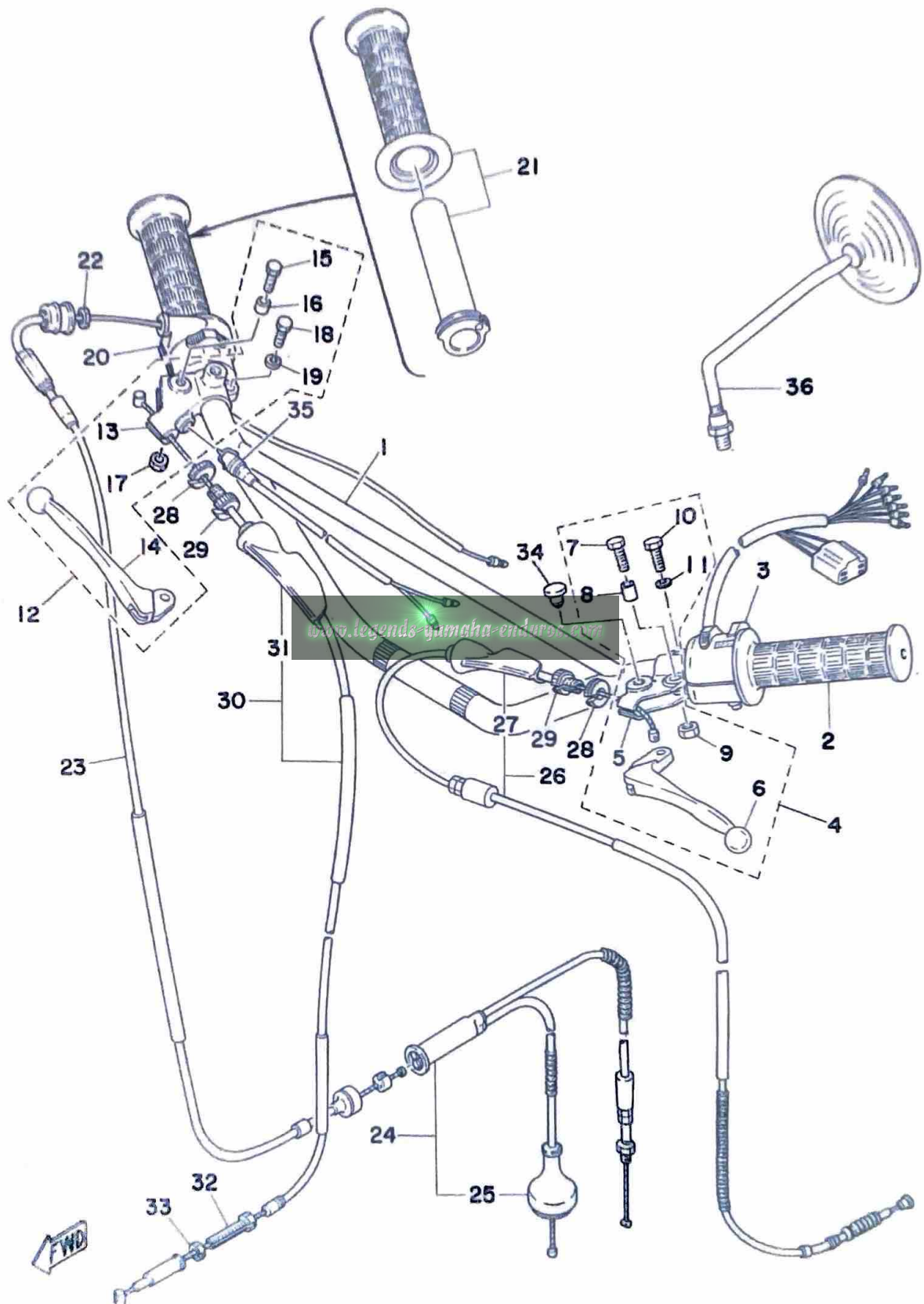
Fig. 20 HANDLE · WIRE
