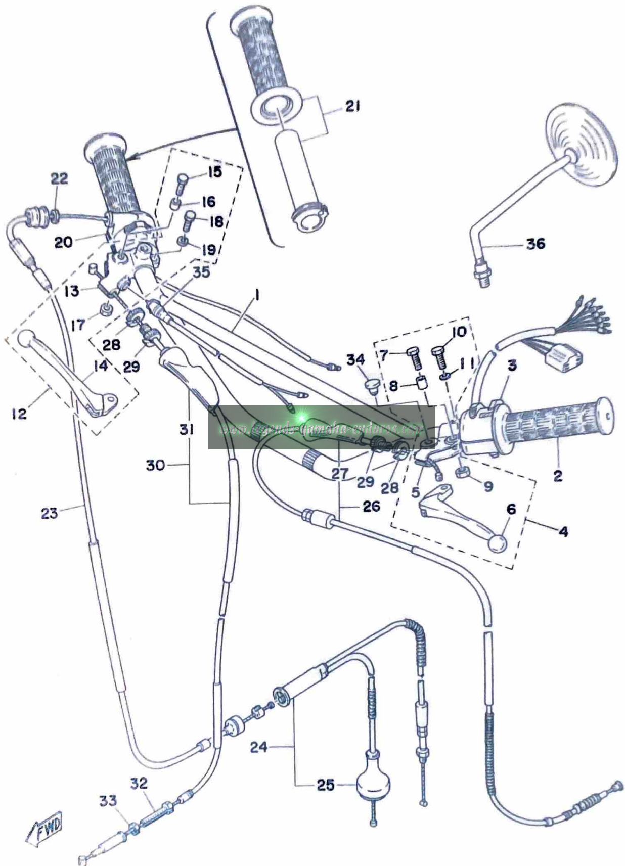
Fig. 20 HANDLE · WIRE
