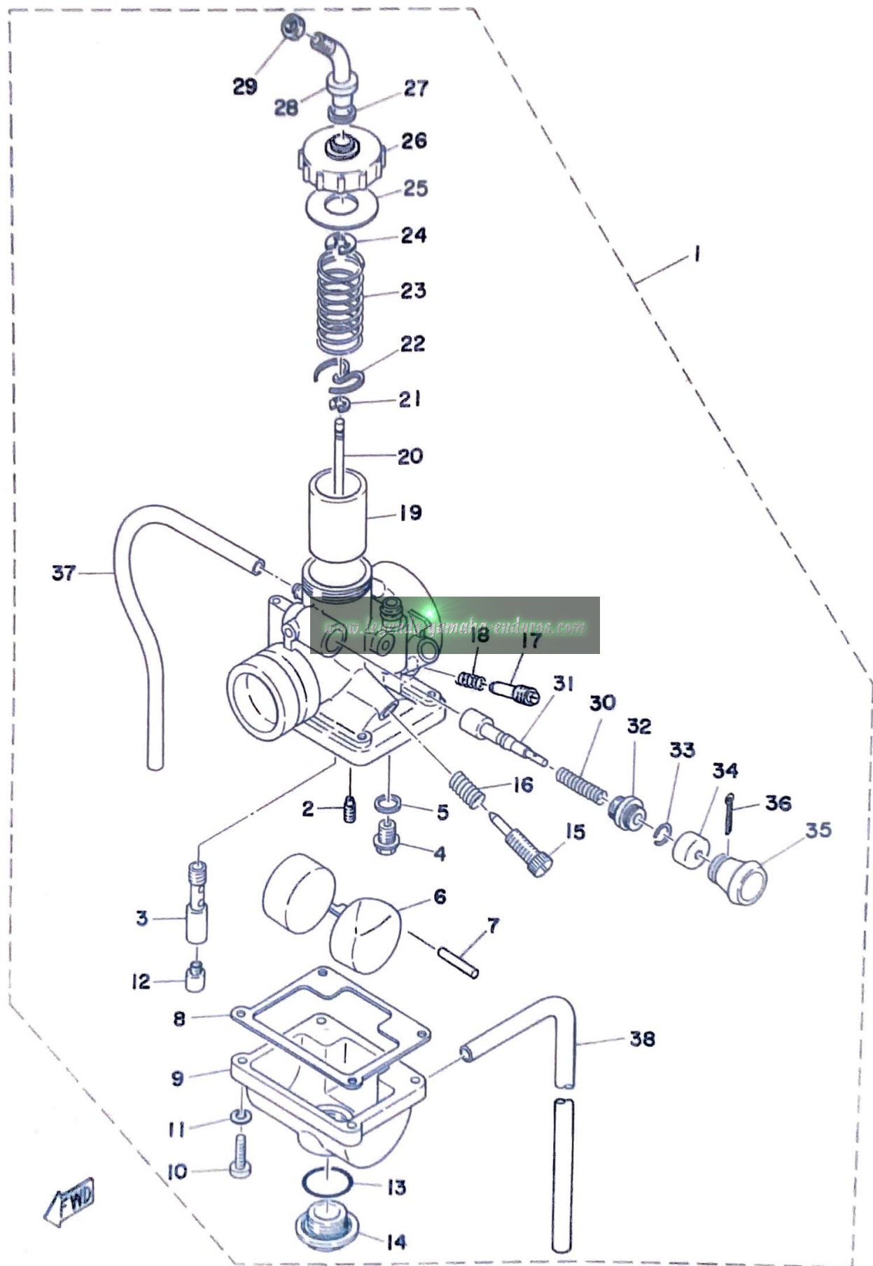
Fig. 10 CARBURETOR
