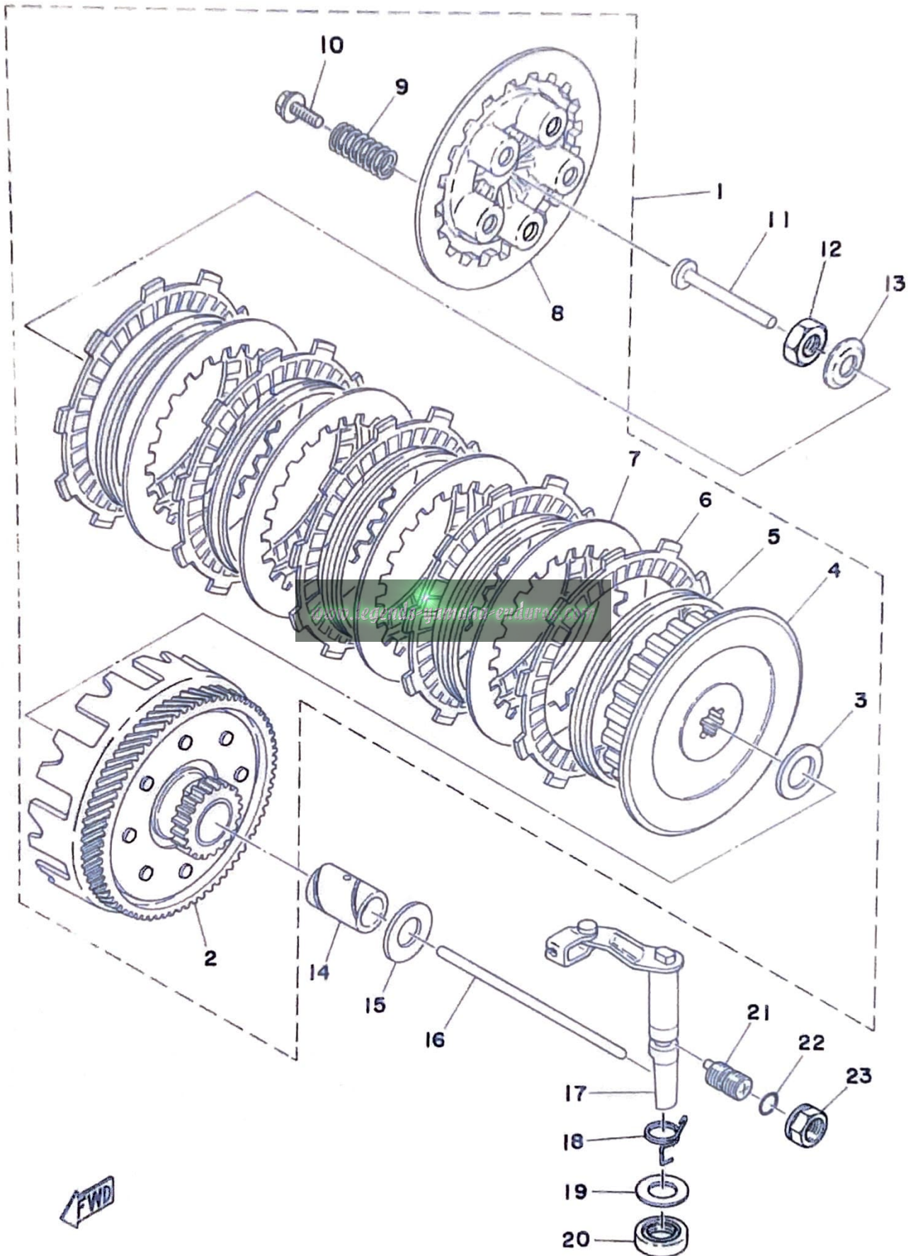
Fig. 4 CLUTCH
