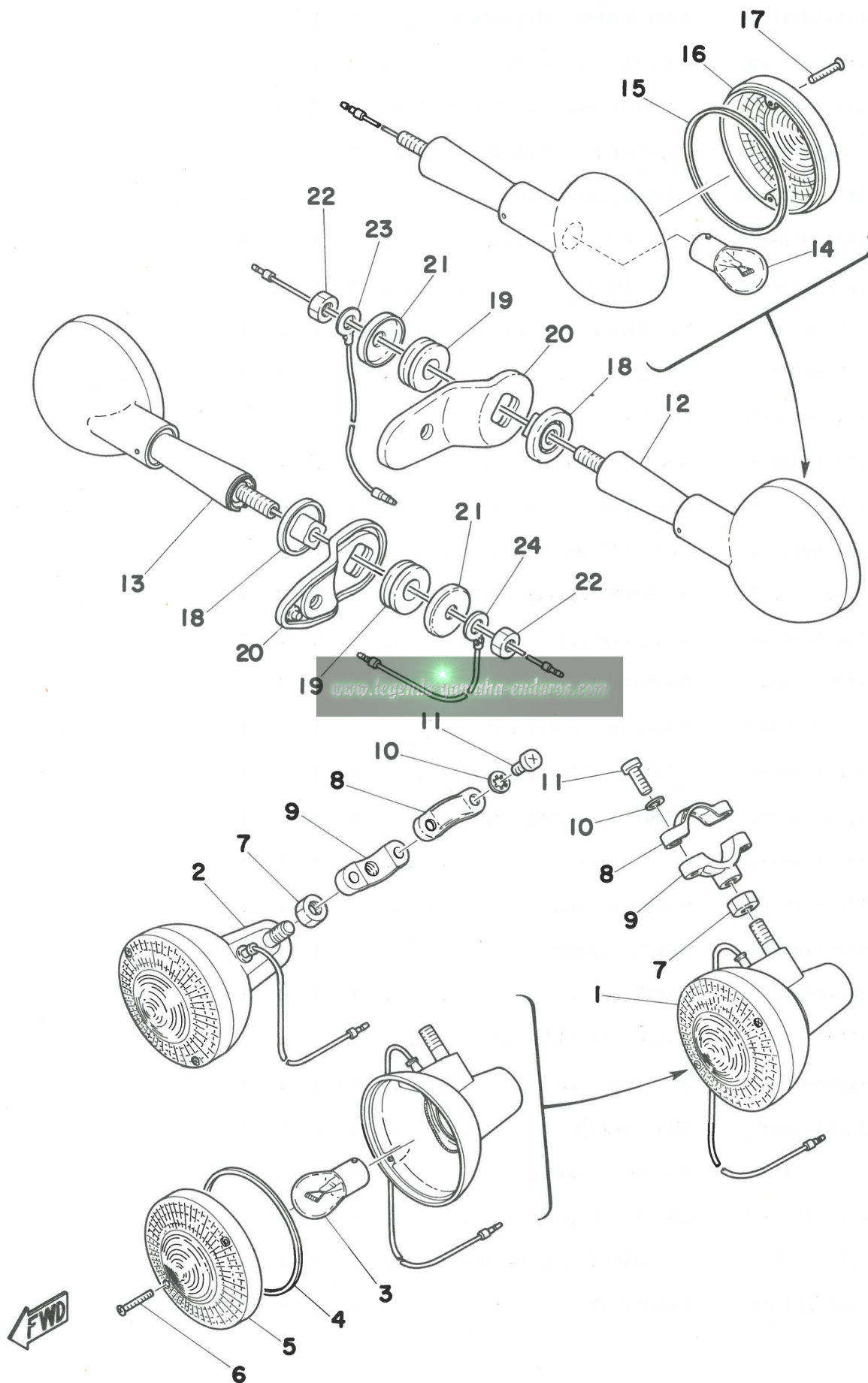
Fig. 34 FLASHER LAMP
