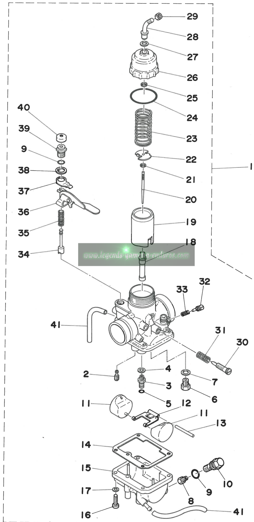
Fig. 13 CARBURETOR(DT250B,DT250C)
