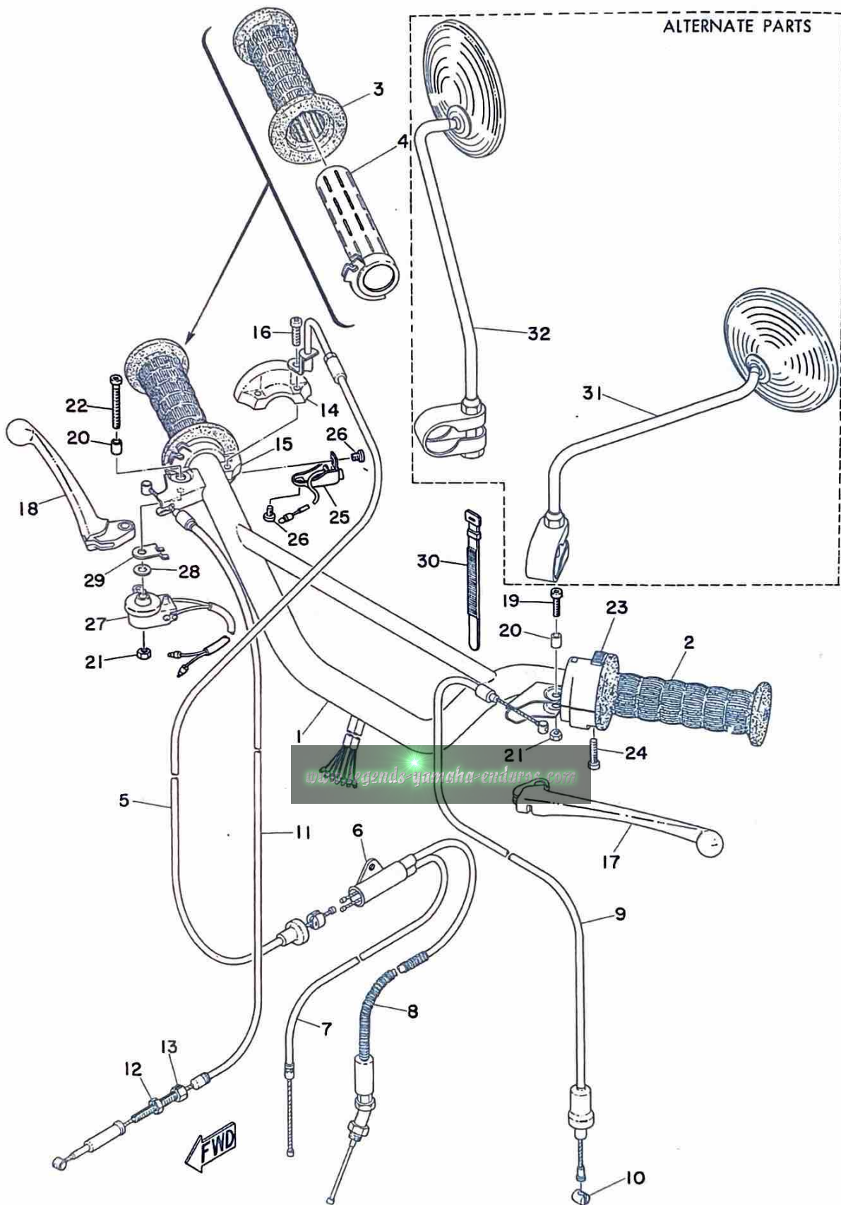
Fig. 20 HANDLE · WIRE
