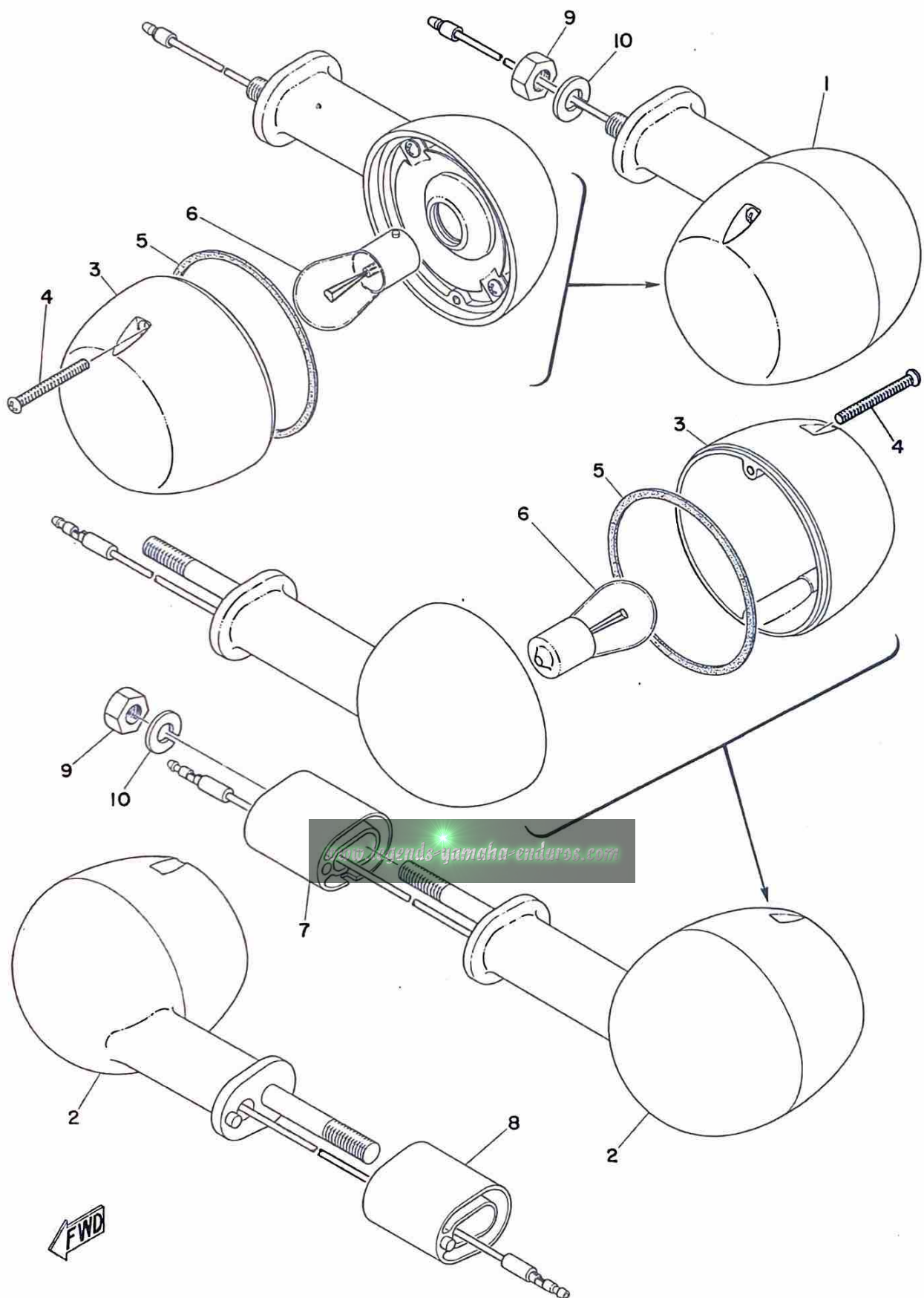
Fig. 28 FLASHER LAMP
