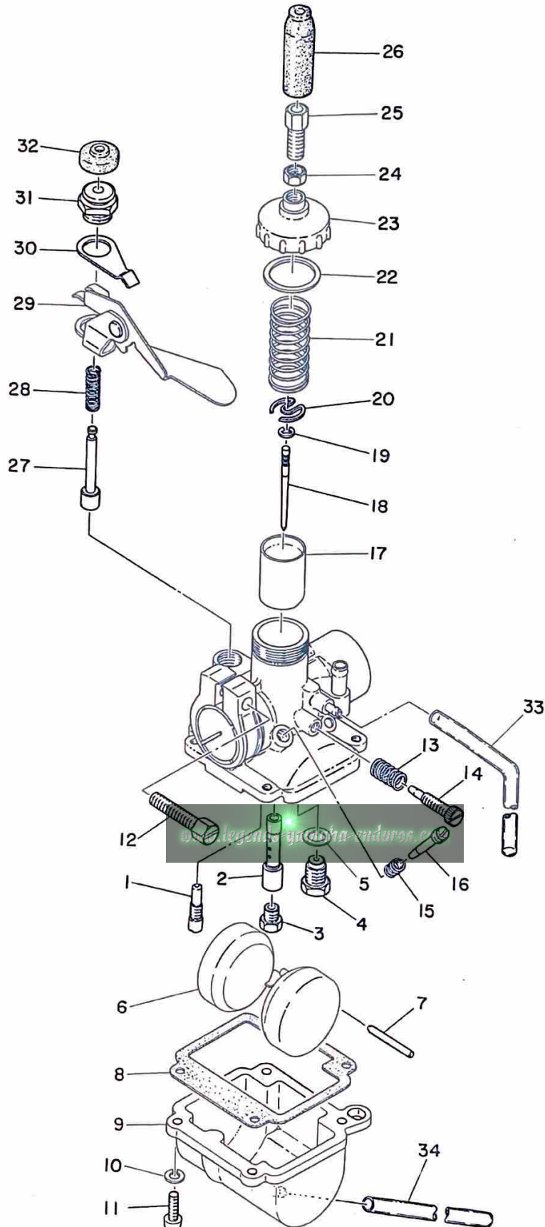
Fig. 10 CARBURETOR
