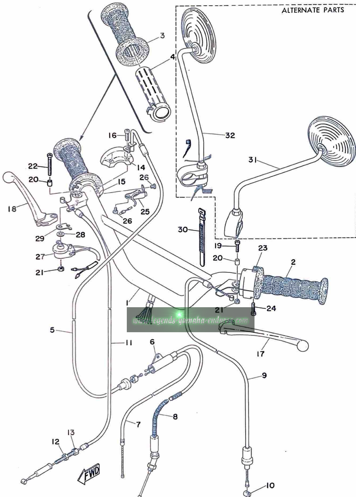
Fig. 20 HANDLE · WIRE
