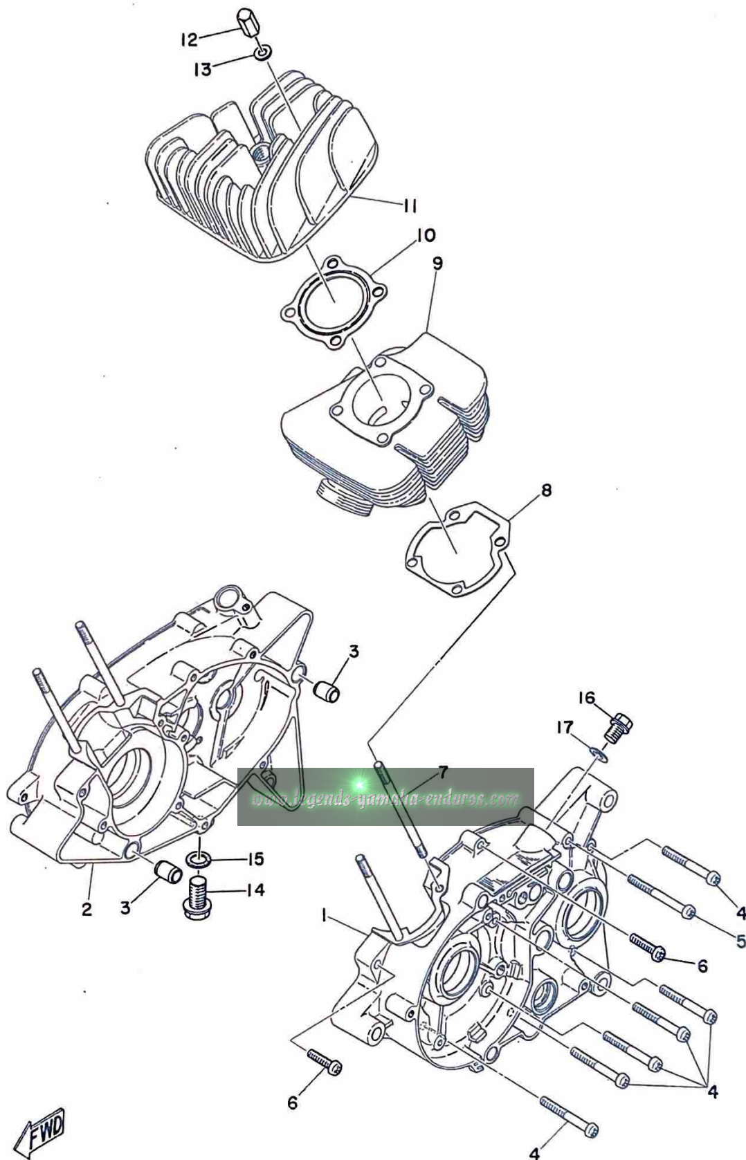
Fig. 1 CRANKCASE · CYLINDER
