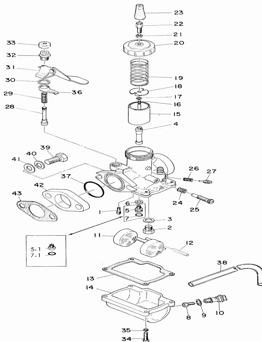
Fig. 11 CARBURETOR
