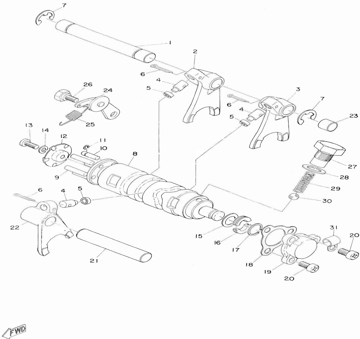
Fig. 6 SHIFTER A
