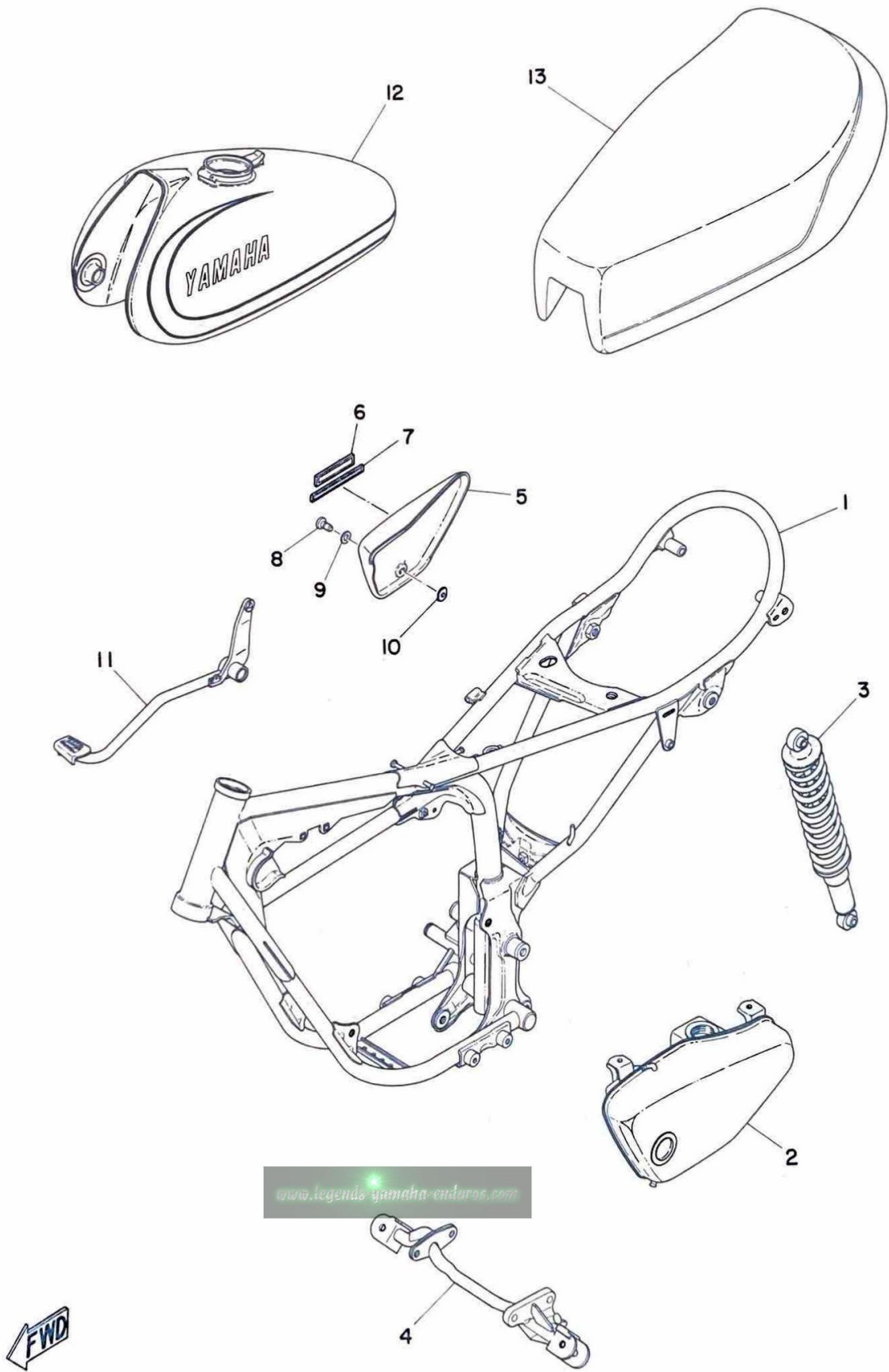
Fig. 6 FRAME · SEAT · REAR CUSHION
