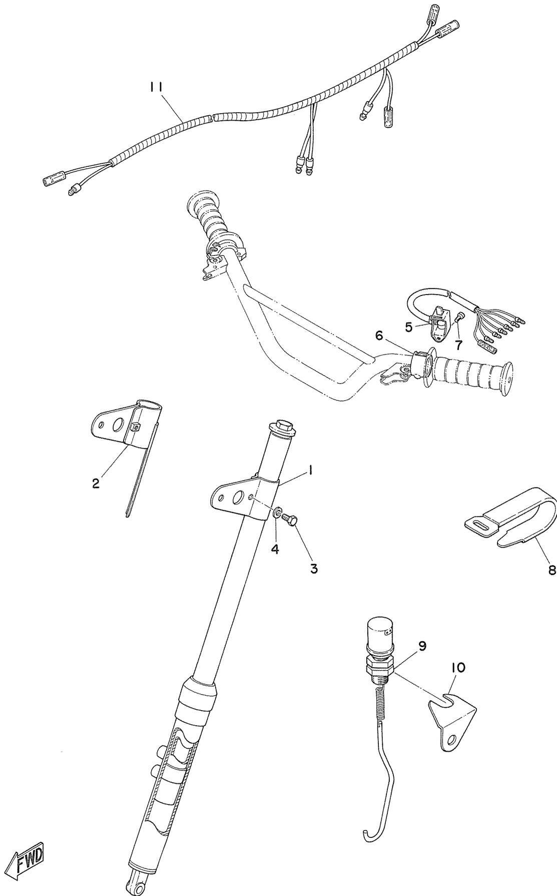
Fig. 27 ELECTRICAL (JT1L)
