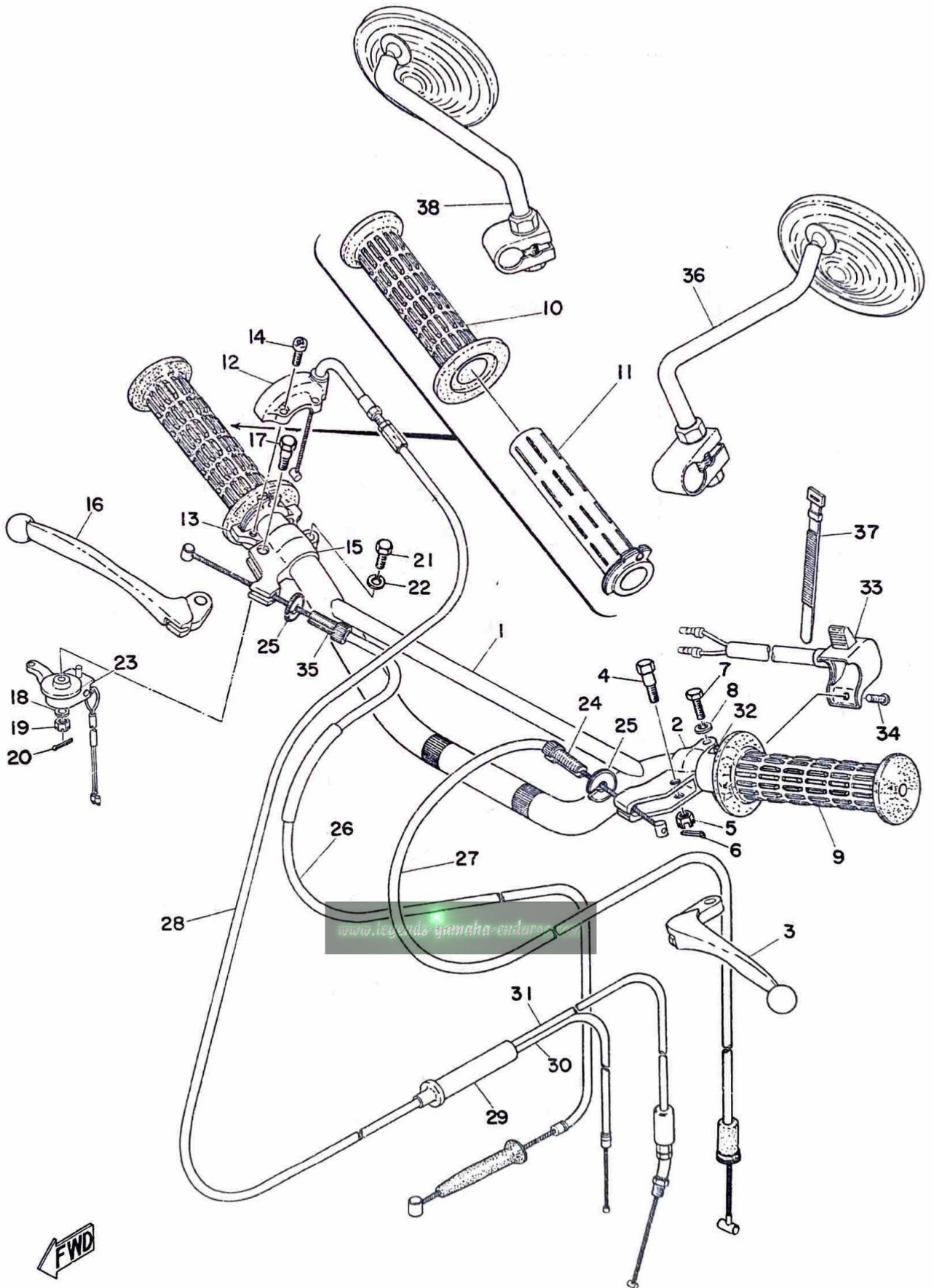
Fig. 18 HANDLE & WIRE
