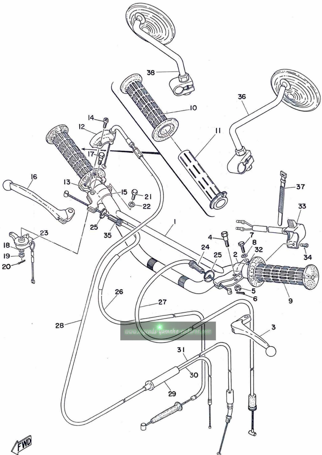
Fig. 18 HANDLE & WIRE
