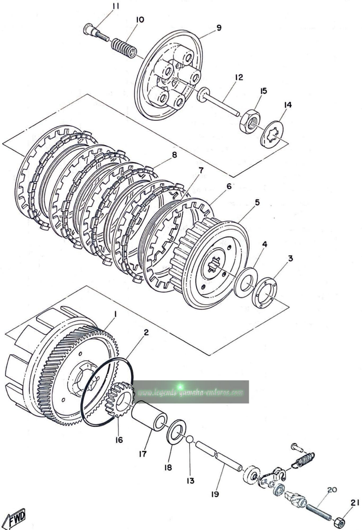
Fig. 4 CLUTCH
