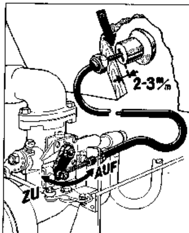
Richtige Einstellung des Start-Vergaser-Zuges
