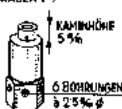
Düsenmodelle und Düsenhöhen zum Soler-Vergaser
