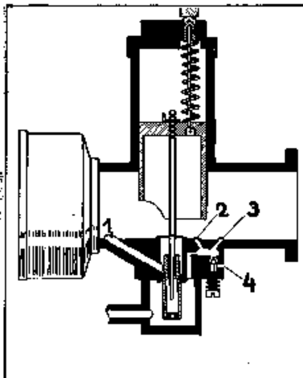
Schematische Zeichnung eines Nachschwenkventils
