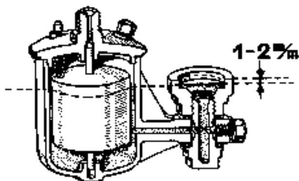
Prüfung des Kraftstoffstandes beim Amal-Vergaser
