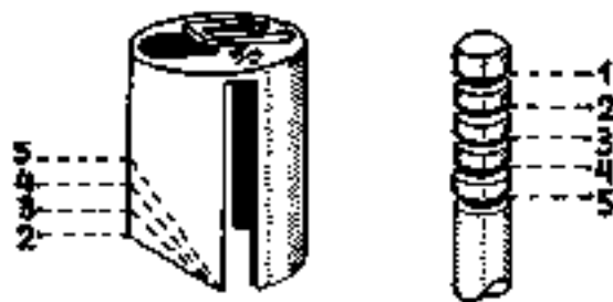
Gasschieberausschnitt und Düsenadelstellungen des Amalg-Vergasers
