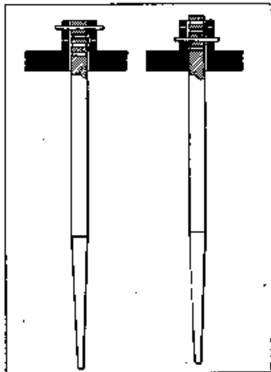
Veränderung der Düsenadelstellung beim Groetzin-Vergaser
