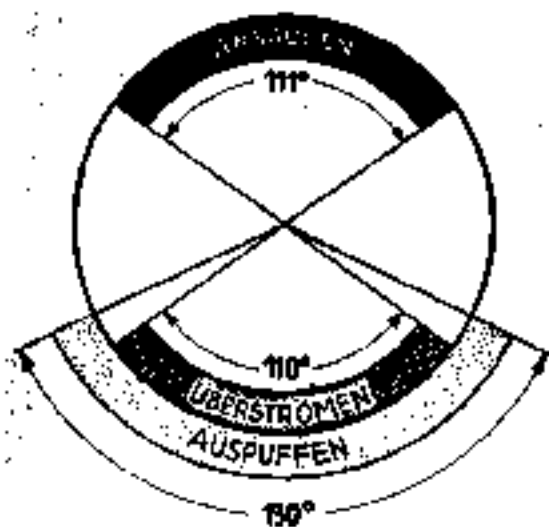
Steuerdiagramm eines Dreikanal-Zweikolbenmotors
