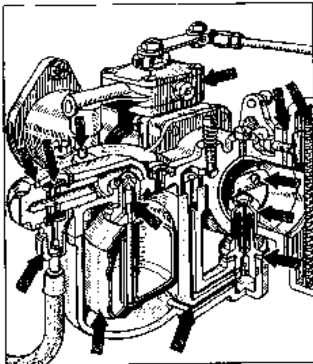
An allen diesen Stellen treten häufig Verschleißerscheinungen bzw. Wartungsfehler (sogenannte mechanische Fehler am Vergaser) auf, die die Vergasereinstellung beeinflussen.
