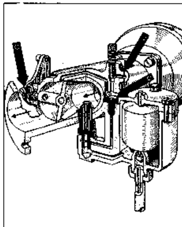
Die drei Einstellfaktoren für den Leerlauf: Leerlauf-Kraftstoffdüse, Leerlauf-Luftstellschraube und Leerlauf-Begrenzungsschraube (Drehmomentbegrenzungsschraube).
