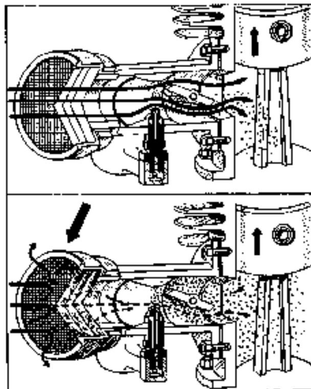
So beeinträchtigt ein verschmutztes Luftfilter die Gemischbildung am Vergaser.
