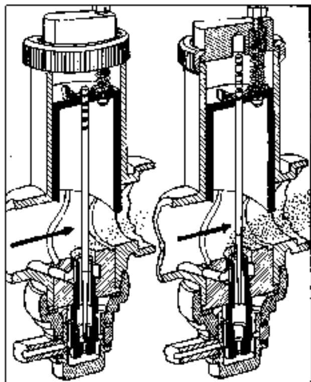
Werkzeuge der konischen Chrennadel: Wird die Nadel im Gasschieber höher gestellt, so wird bei gleicher Gasschieberstellung das Gemisch reicher und ungefährt.
