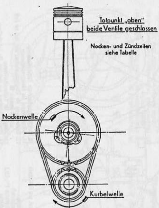
Ventil- und Zündungs-Einstellung
