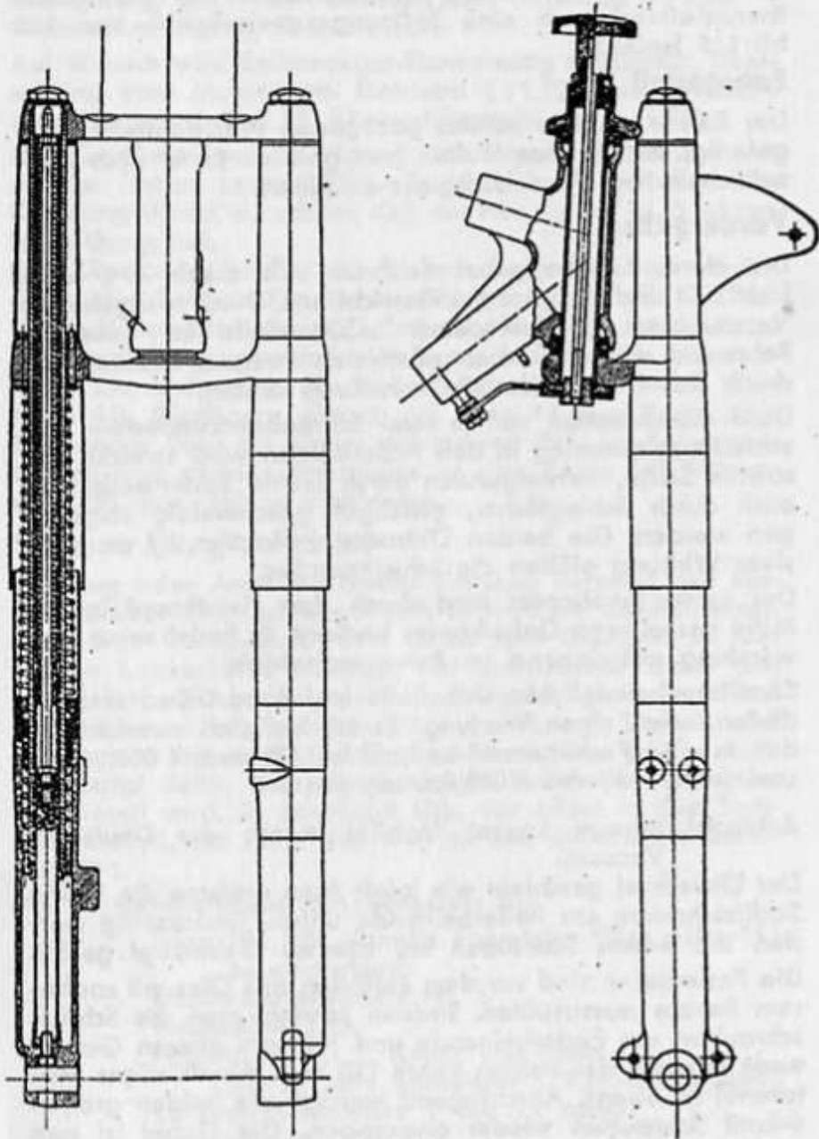
Horex-Teleskopgabel
