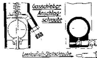
Abb. 24. Amal-Vergaser im Schnitt.
