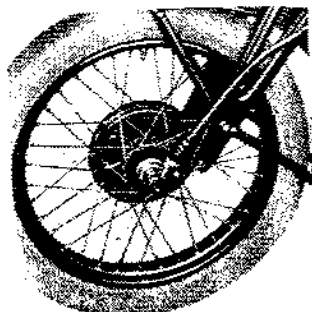
Abb. 42. Demontage des Vorderrades u. Tachometerantriebes: Man löst die beiden Achsmutter und öffnet die eine Gabelscheide vorsichtig etwas m. dem Schlüssel. Um den Tachometerantrieb zu lösen, braucht man nur den Sperrknopf einzudrücken und kann dann das Kabel herausziehen. Bei Wiedereinsetzen ist darauf zu achten, daß die Kabelführungszunge richtig in die Antriebsführung eingesetzt wird.
