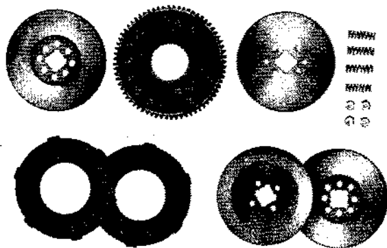
Abb. 18. Kupplung in Einzelteile zerlegt: Oben in der Mitte die zentrale Antriebscheibe, links darunter die beiden Belaglamellen (Kork bzw. Jurid), daneben die entsprechenden Stahlscheiben. Die gesamte Kupplung arbeitet im Ölbad.
