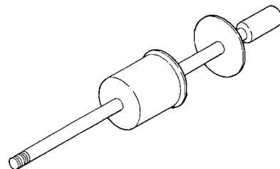
09930-30102 Rotor remover sliding shaft Axe de glissement d'arrache-rotor
