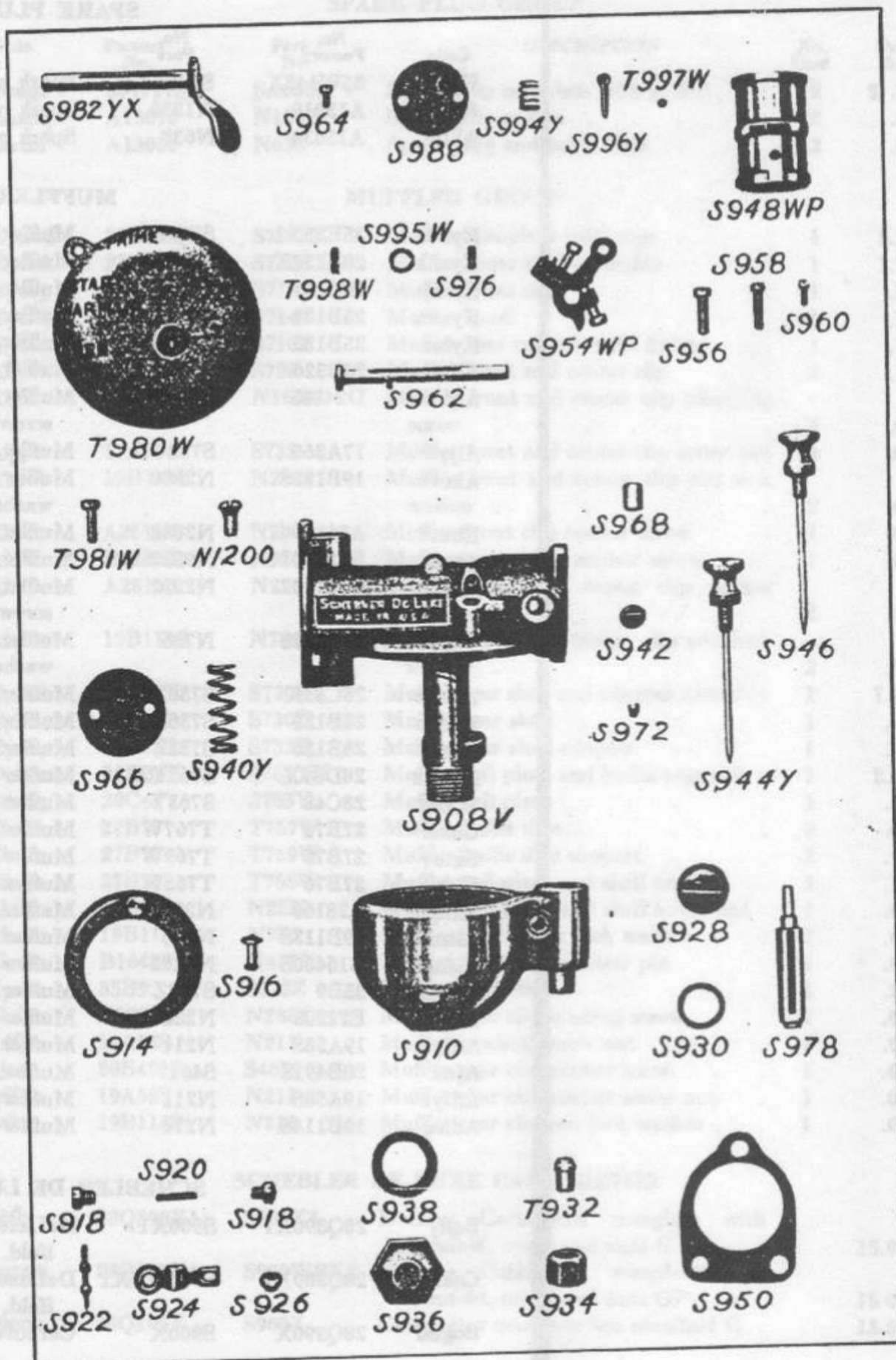
De Luxe Carburetor Group
