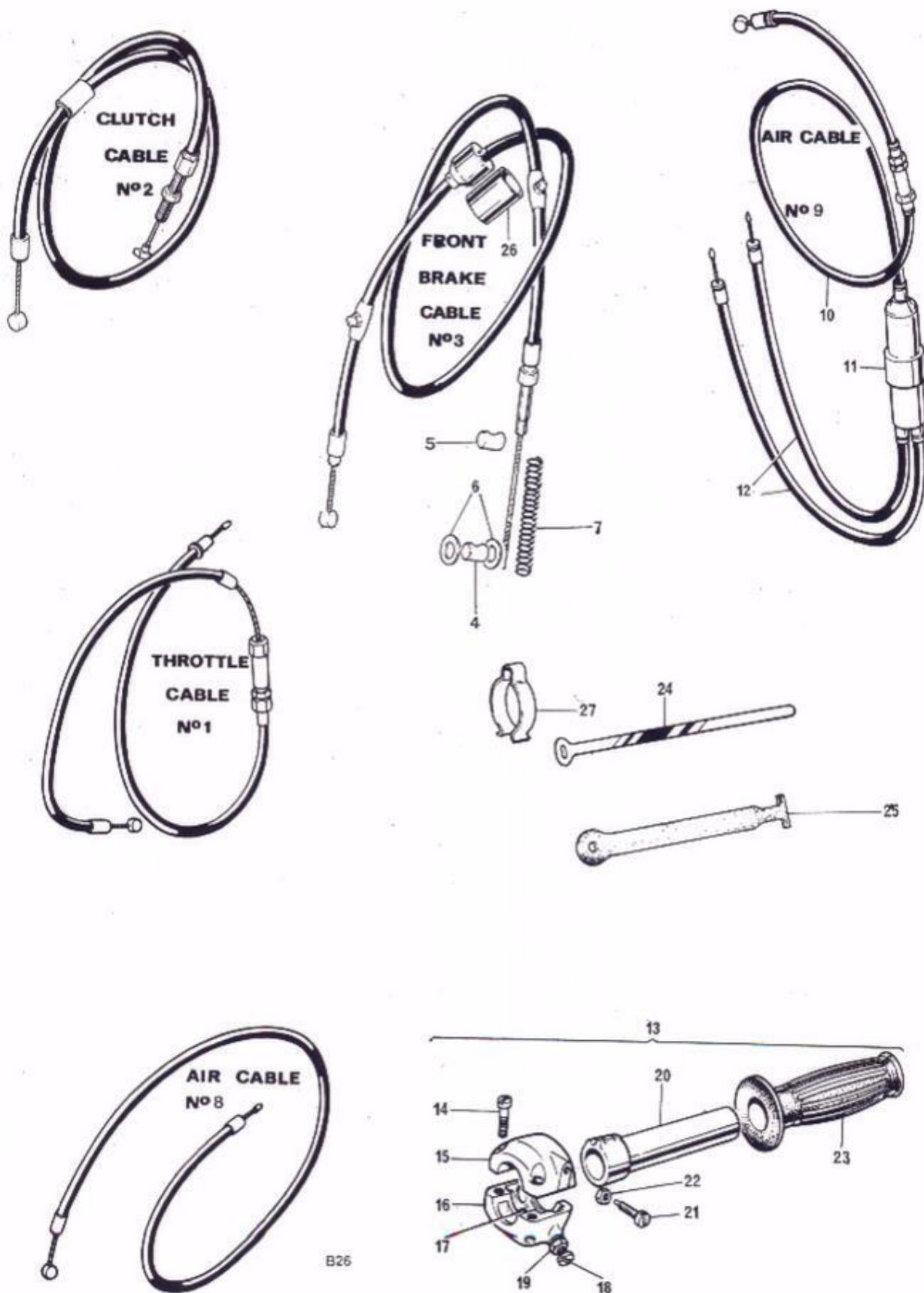
Fig. 27. CONTROL CABLES
