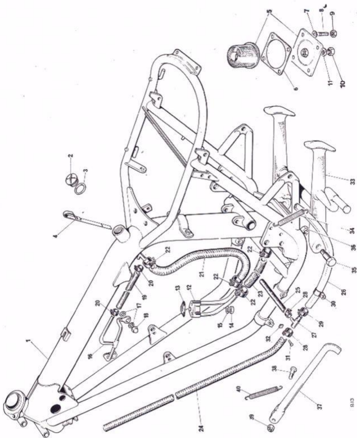
FIG. 14. FRAME
