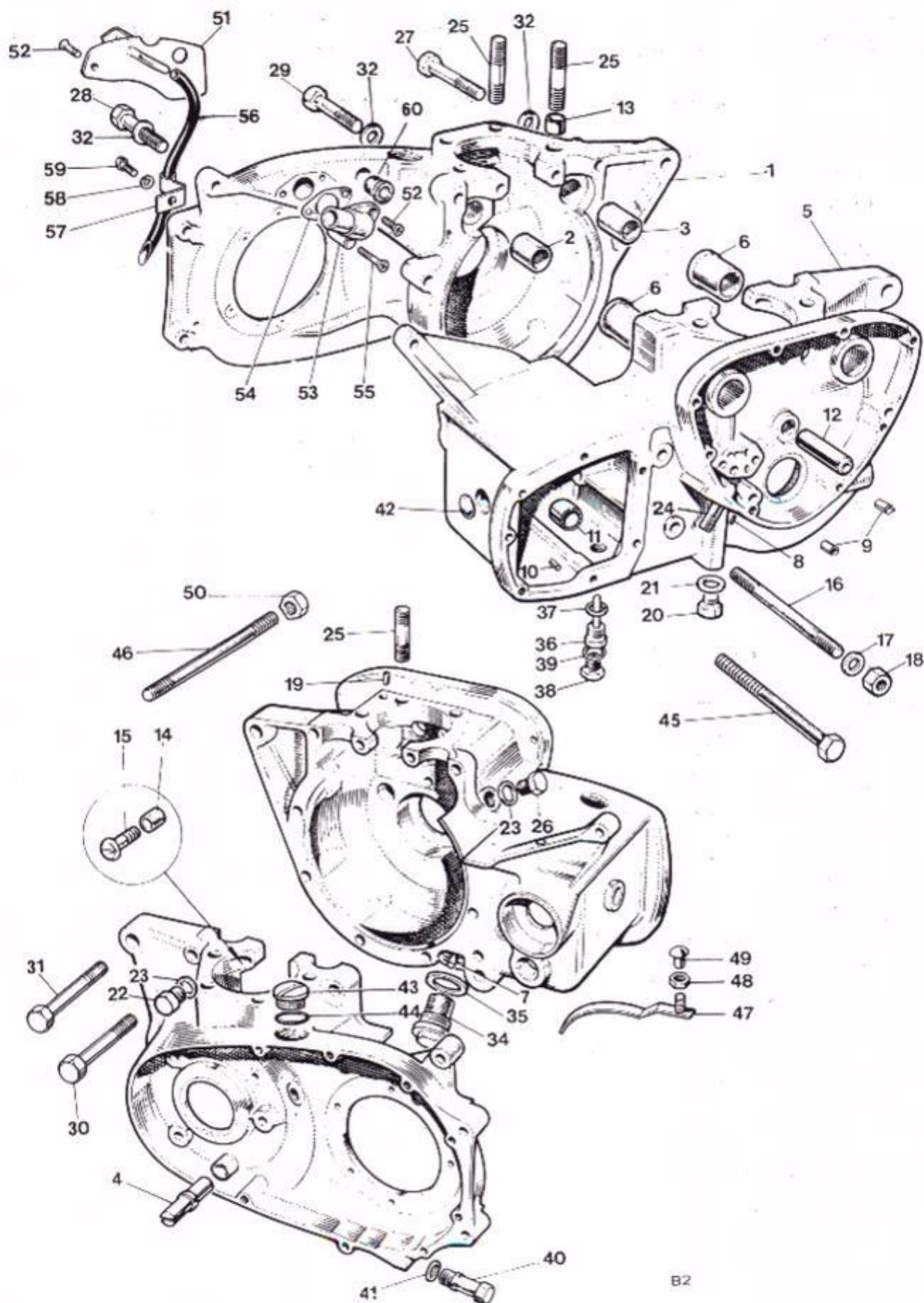
Fig. 2. CRANKCASE
