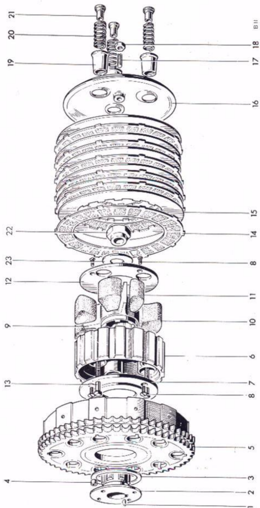
Fig. 12. CLUTCH
