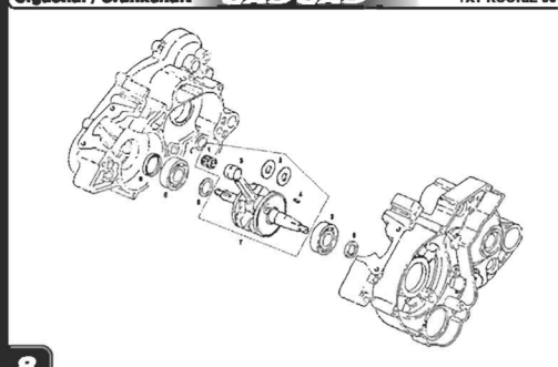
Cigüeñal / Crankshaft
