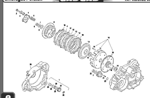
Embrague / Clutch
