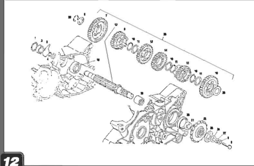
Eje secundario / Counter shaft
