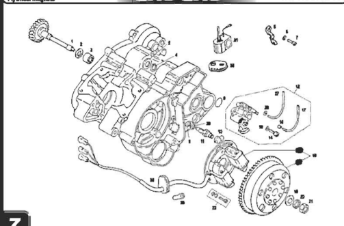
Volante magnético / Flywheel magnet
