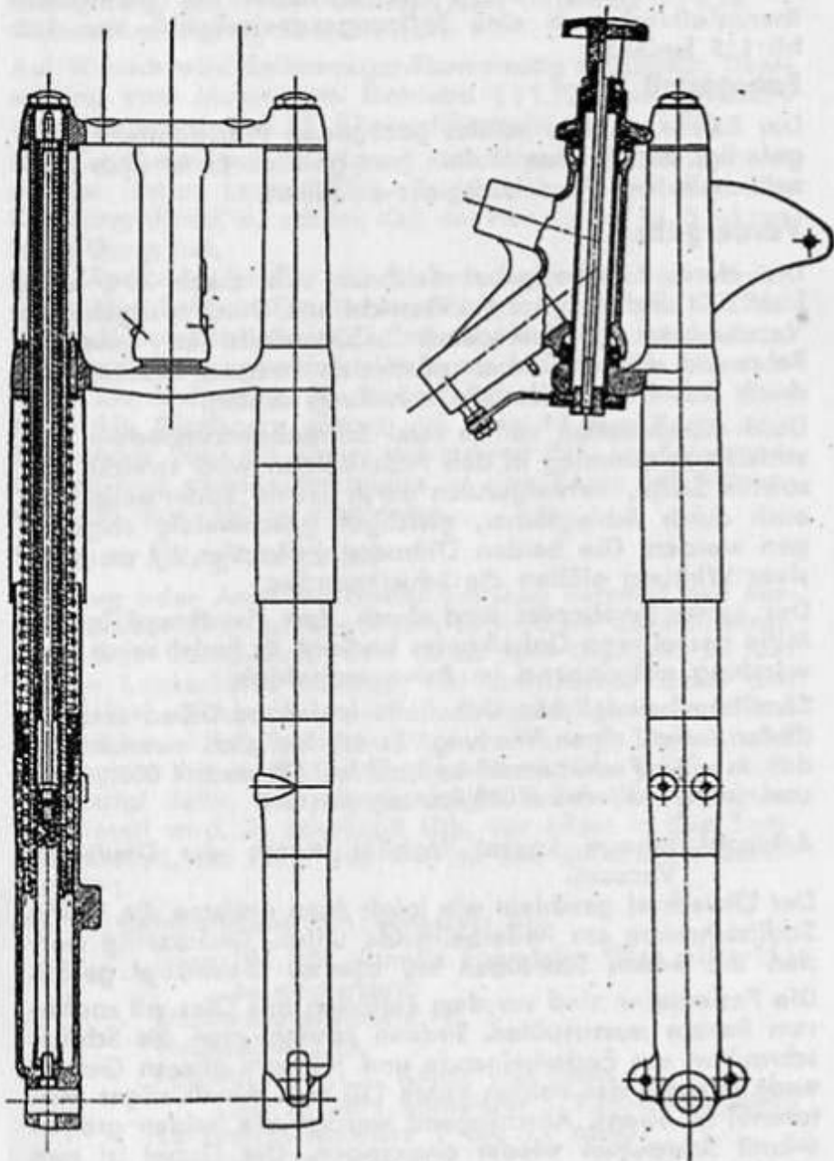
Horex-Teleskopgabel
