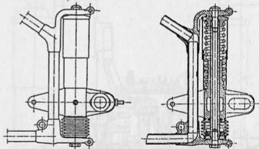
Schnittbild d. Hinterrad-Federung
