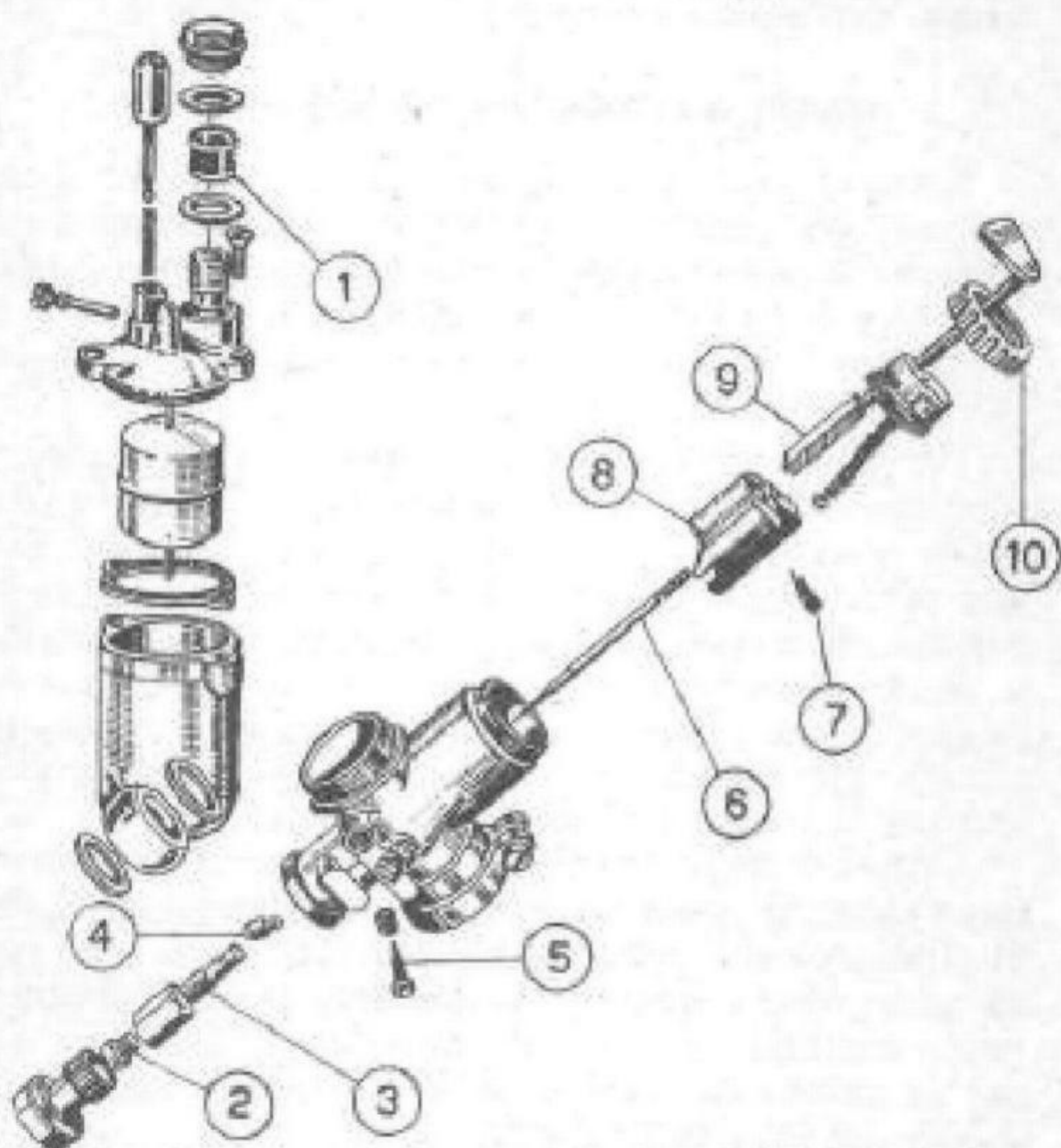
Fig. 12 — Carburatore smontato per la pulizia: 1) Filtro del carburatore - 2) Getto principale (o del massimo) - 3) Polverizzatore portagetto - 4) Getto del minimo - 5) Vite regolazione aria minima - 6) Spillo conico - 7) Malletta fissaggio spillo conico - 8) Valvola del gas - 9) Tegolo dello starter - 10) Chiusura di chiusura.
