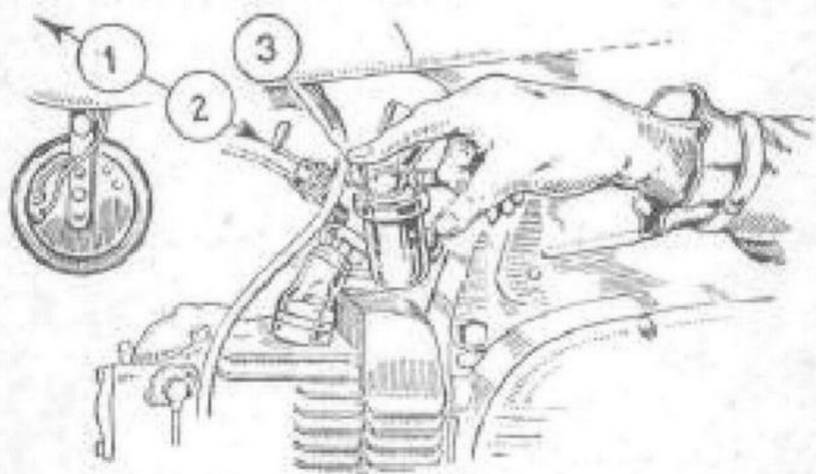
Fig. 3 — Starter e agitatore collegante sul carburatore: 1) Starter in posizione di marcia - 2) Starter in posizione di avviamento - 3) Agitatore.
