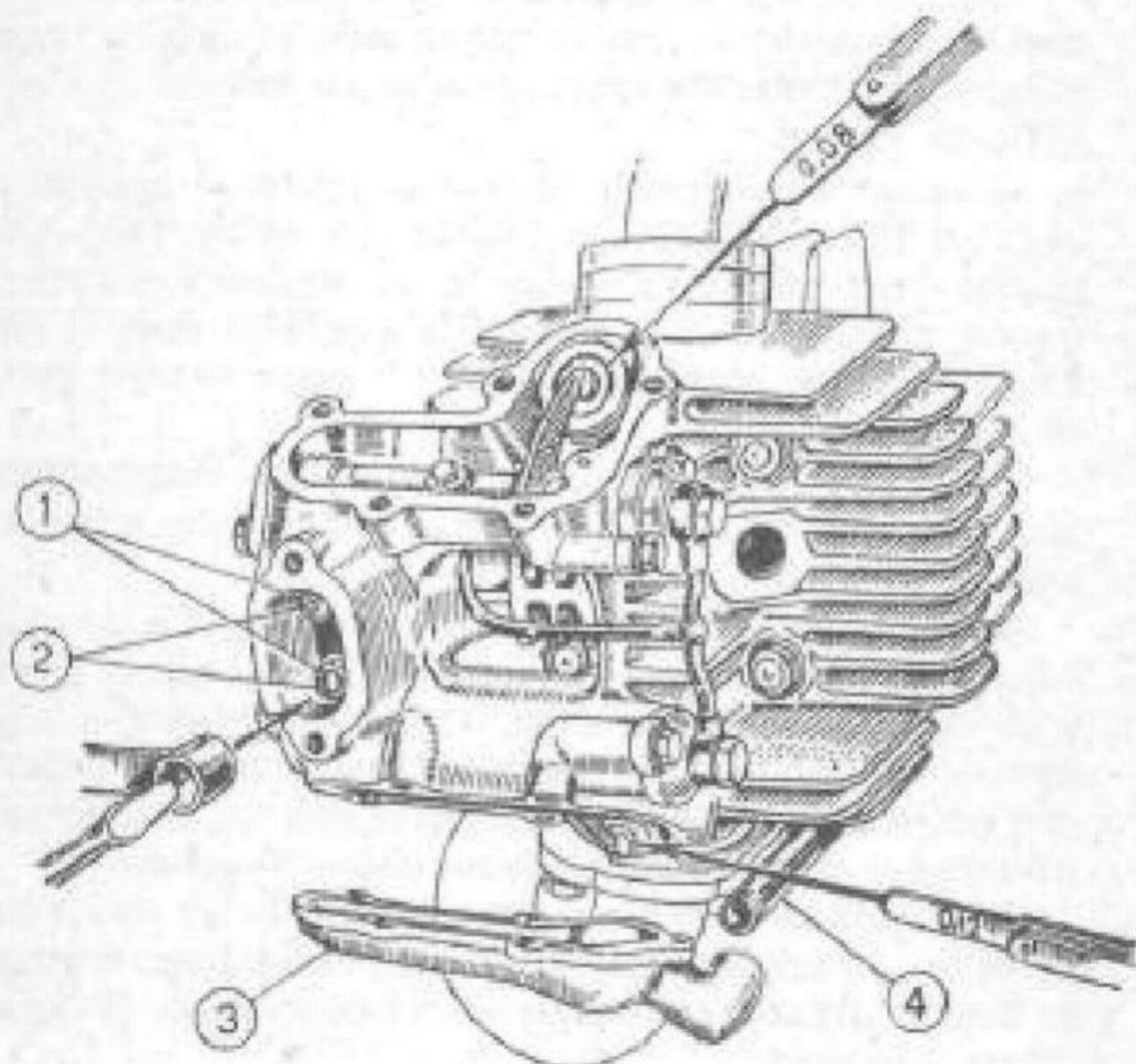
Fig. 13 — Regolazione giuoco comando valvole: 1) Viti di regolazione - 2) Controdadi - 3) Coperchio valvola scarico con raccogliatore olio - 4) Tubo recupero olio dai bilancieri.
