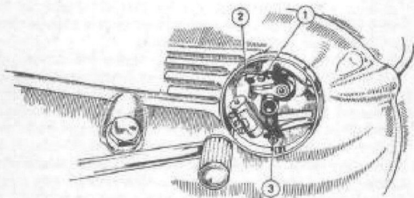
Fig. 14 — Regolazione contatti ruttore: 1) Vite bloccaggio contatto fisso - 2) Tacche per appoggio cacciavite - 3) Viti a colonnetta fissaggio piastra ruttore e coperchio esterno.
