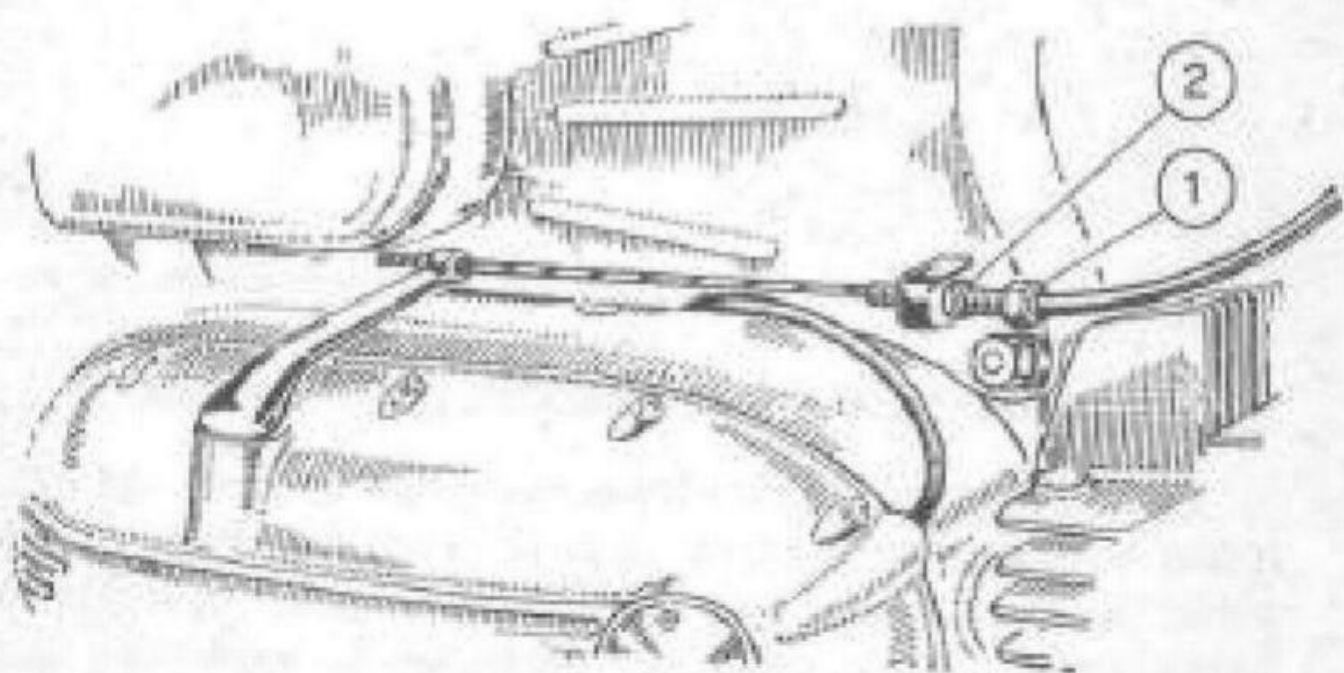
Fig. 11 — Regolazione comando frizione: 1) Tenditore della trasmissione flessibile - 2) Controdado.
