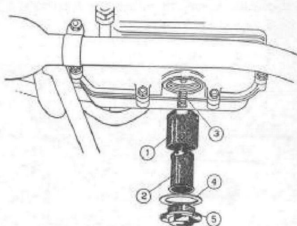
Fig. 6 — Filtro della pompa di mandata olio: 1) Filtro esterno - 2) Filtro interno - 3) Molla ritegno filtri - 4) Guarnizione del tappo - 5) Tappo scarico olio.
