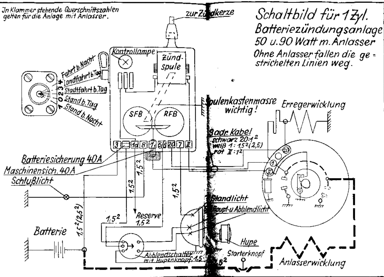
Abb. 51. Elektrisches Schaltbild der Zylinder-Anlagen.
