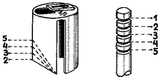
Gasschieberausschnitte und Düsenadelstellungen des Amal-Vergasers
