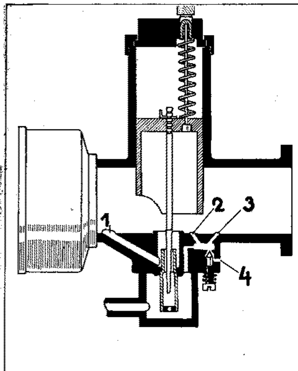
Schematisches Bild eines Nadeldüsenvergaser
