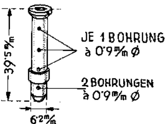
Düsenmodelle und Düsenhütchen beim Solex-Vergaser
