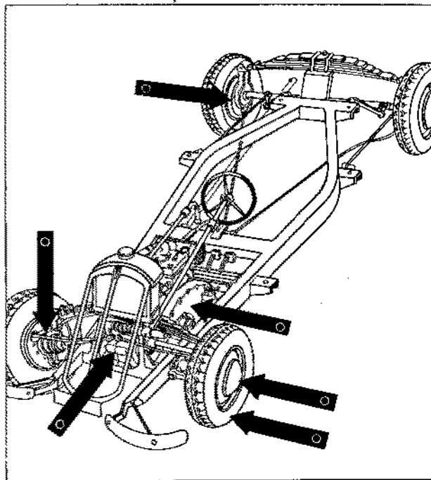
An den angegebenen Stellen kann durch vernachlässigte Wartung ein erhöhter Eigenkraftbedarf des Fahrzeuges entstehen, der den Kraftstoffverbrauch erhöht.
