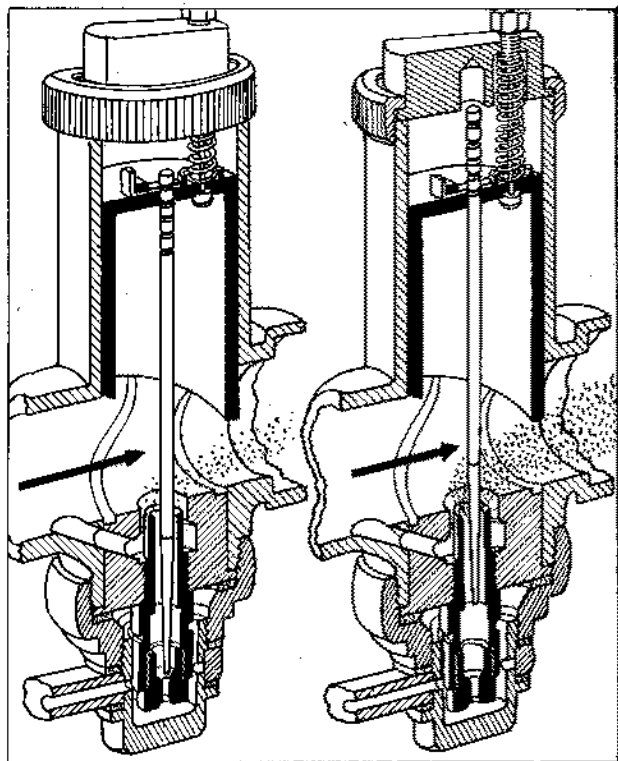
Wirkungsweise der konischen Düsennadel: Wird die Nadel im Gasschieber höher gesetzt, so wird bei gleicher Gasschieberstellung das Gemisch reicher und umgekehrt.
