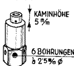
Düsenmodelle und Düsenhütchen beim Solex-Vergaser
