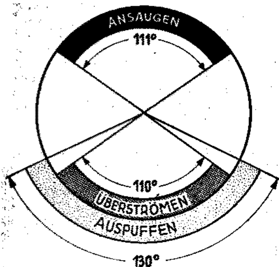
Steuerdiagramm eines Dreikanal-Zweitaktmotors
