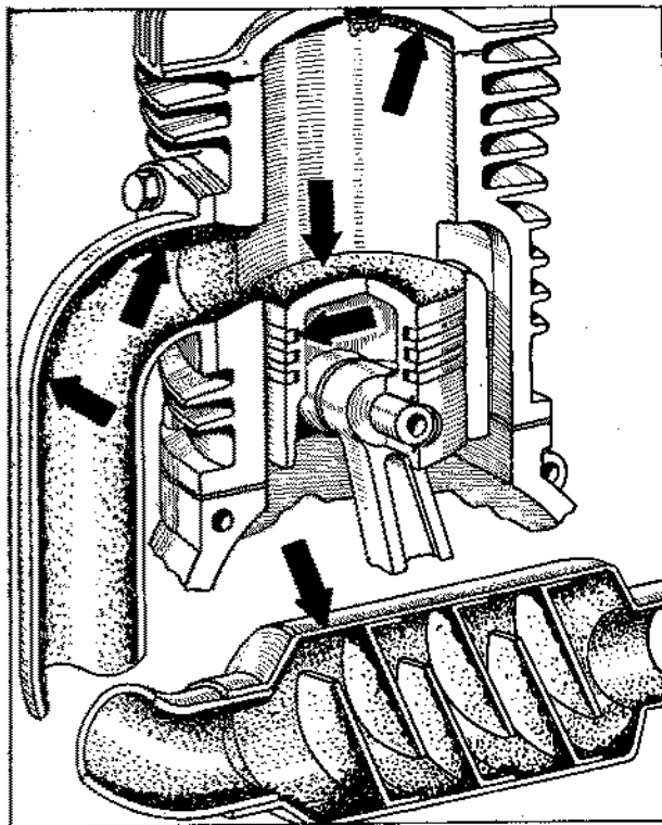
Rückstandsbildung im Motor, die den Verbrennungsablauf und damit Leistung und Verbrauch des Motors ungünstig beeinflusst: im Zylinderdeckel, auf dem Kolbenboden, in den Kolbenringnuten, in den Auslaßschlitzen, in Auspuffrohr und Auspuffkopf.
