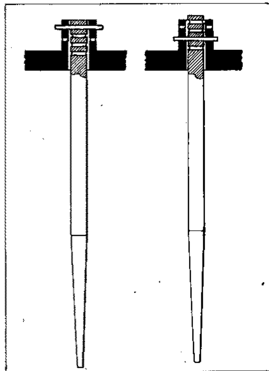
Veränderung der Düsennadelstellung beim Graetzin-Vergaser
