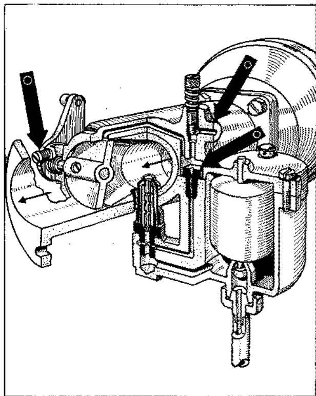
Die drei Einstellfaktoren für den Leerlauf: Leerlauf-Kraftstoffdüse, Leerlauf-Luftstellschraube und Leerlauf-Begrenzungsschraube (Drosselanschlagschraube).
