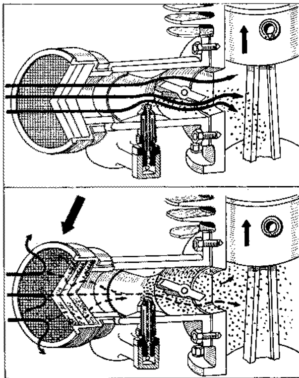
So beeinflusst ein verschmutztes Luftfilter die Gemischbildung im Vergaser.
