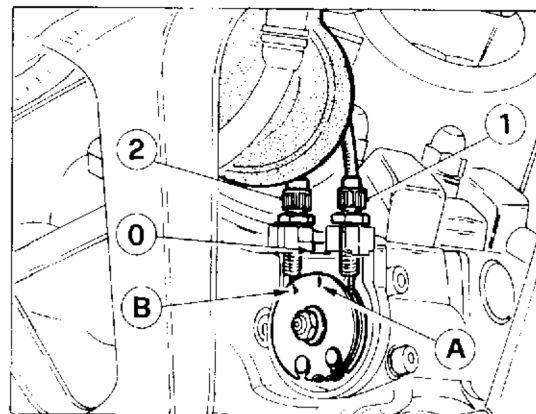
1, 2) Élément de réglage / Steilschraube / Registro 0) Indice fixe sur le couvercle / Fixanzeige am Deckel / Indice fijo s/tapa A, B) Indice sur la poulie / Anzeige an der Scheibe / Indico s/polea
