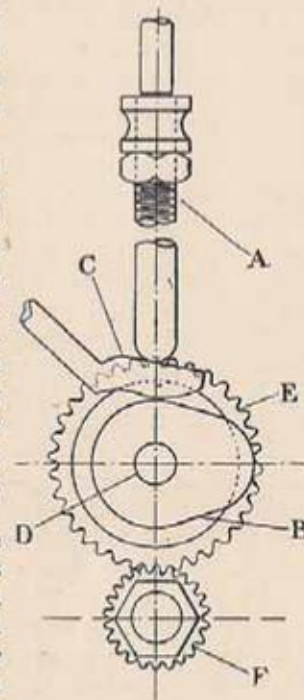
FIG. 27. CAM VALVE ACTION
