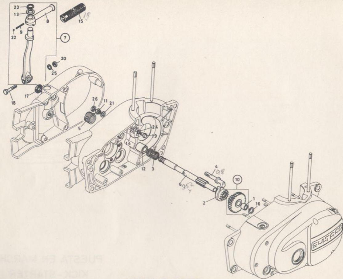
PUESTA EN MARCHA KICK-STARTER
