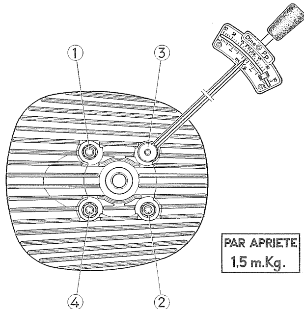
Fig. 16. — Culata: Orden a seguir en el apriete
