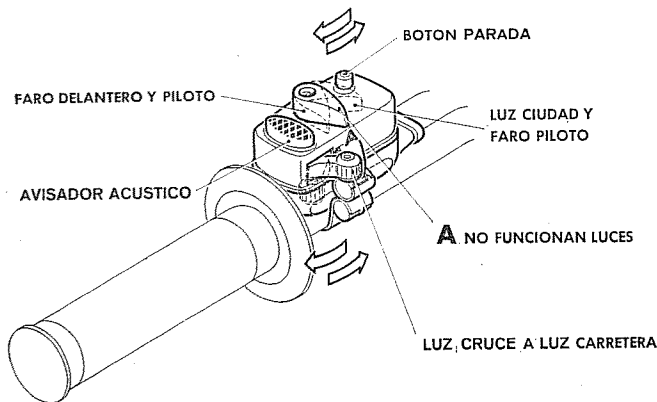
Fig. 5. — Interruptor-conmutador.
