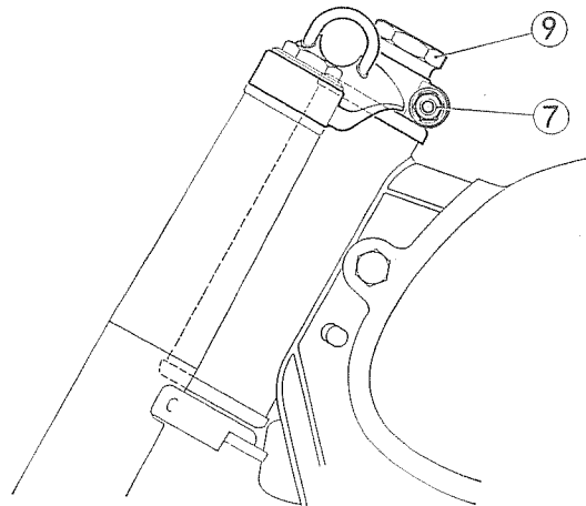
Fig. 21. — Reglaje del juego de la dirección.
