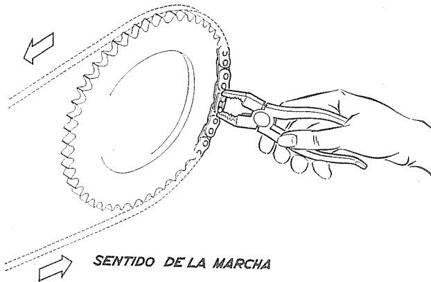
Fig. 20. — Cadena secundaria: Montaje y desmontaje del eslabón-enganche y posición del clip con relación al sentido de la marcha.
