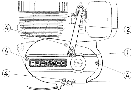
Fig. 12. — Desmontaje del cárter exterior lado volante.
