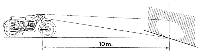
Fig. 15. — Reglaje del faro delantero.
