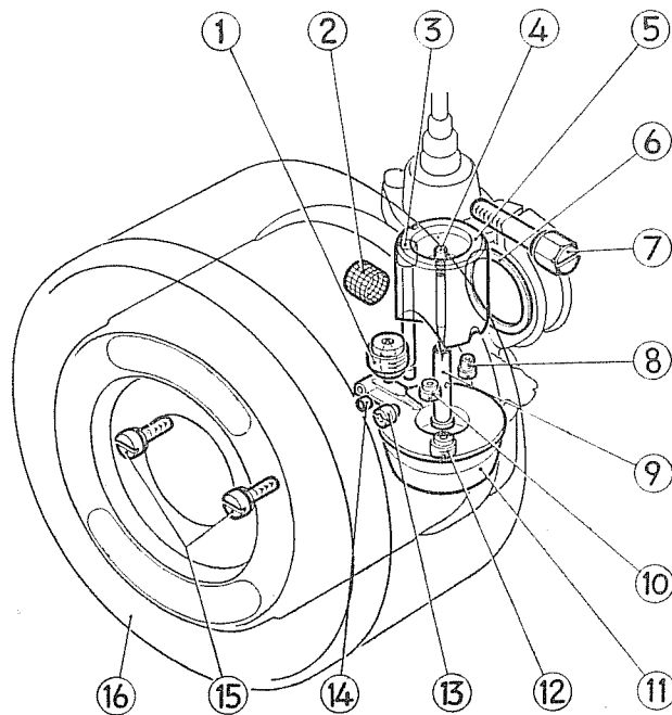
Fig. 32. — Carburador ZENITH: Limpieza e inspección.
