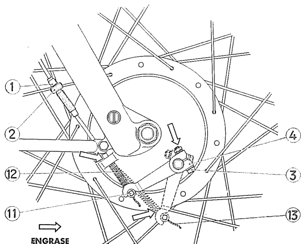
Fig. 26. — Freno delantero: Reglaje, recuperación desgaste y engrase.
