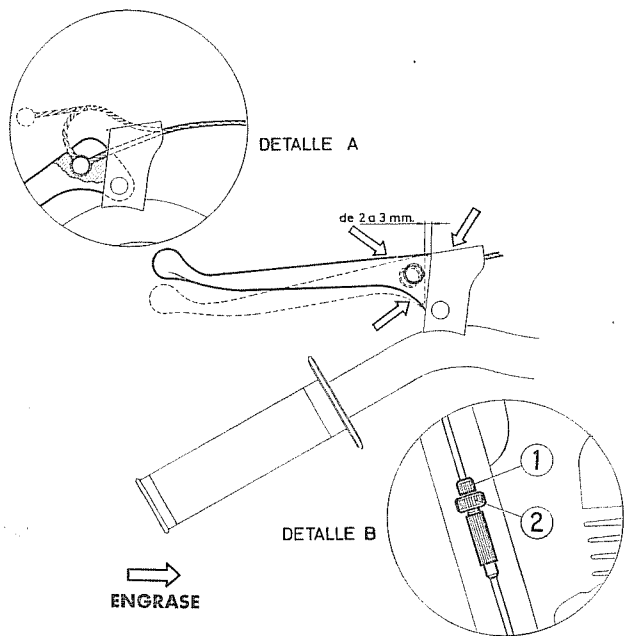
Fig. 29. — Mando embrague: Reglaje, engrase y cambio de cable.
