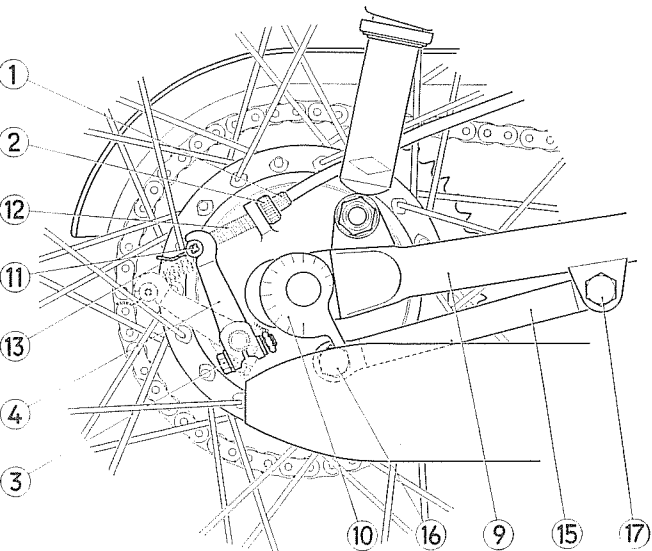
Fig. 27.— Freno trasero: Recuperación desgaste y engrase.
