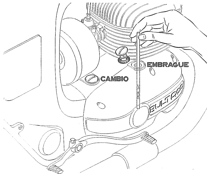
Fig. 17. — Niveles cambio y embrague.
