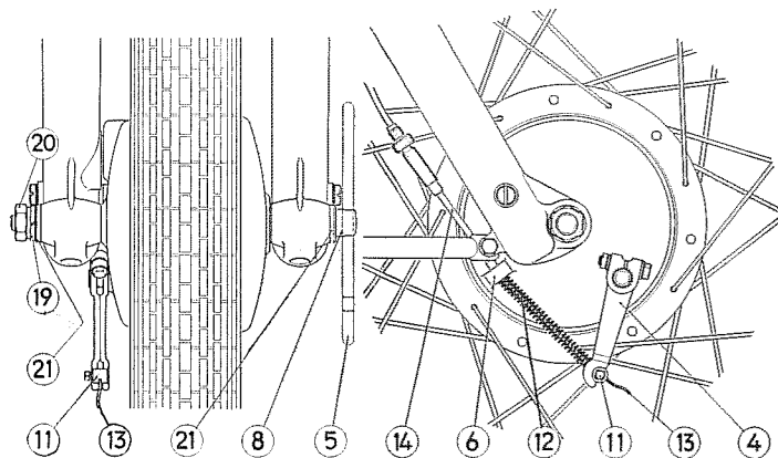
Fig. 22. — Rueda y freno delantero.
