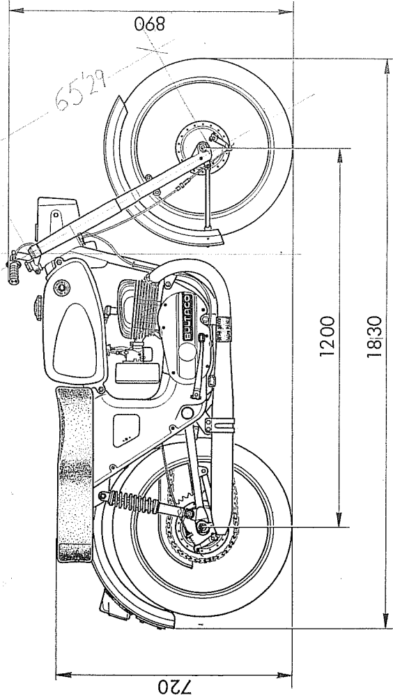
Fig. 35. — Dimensiones principales.
