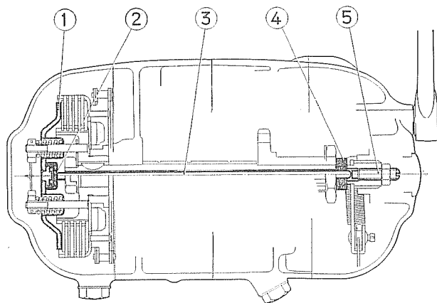
Fig. 28.— Esquema embrague.
