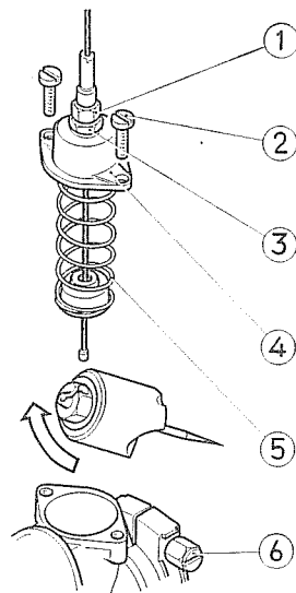
Fig. 34. — Cambio cable gas.
