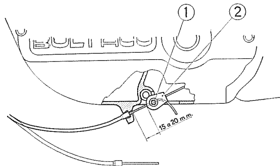
Fig. 30. — Cambio de cable embrague.
