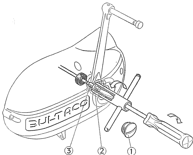
Fig. 31.—Reglaje de la varilla de embrague.
