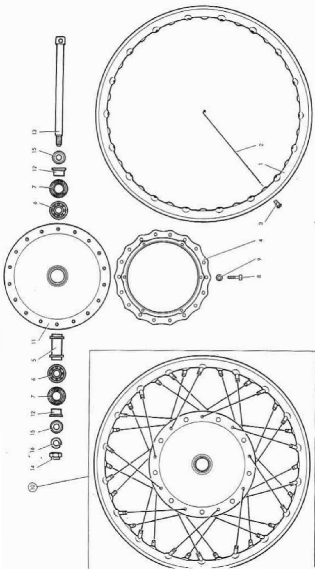
RUEDA DELANTERA
