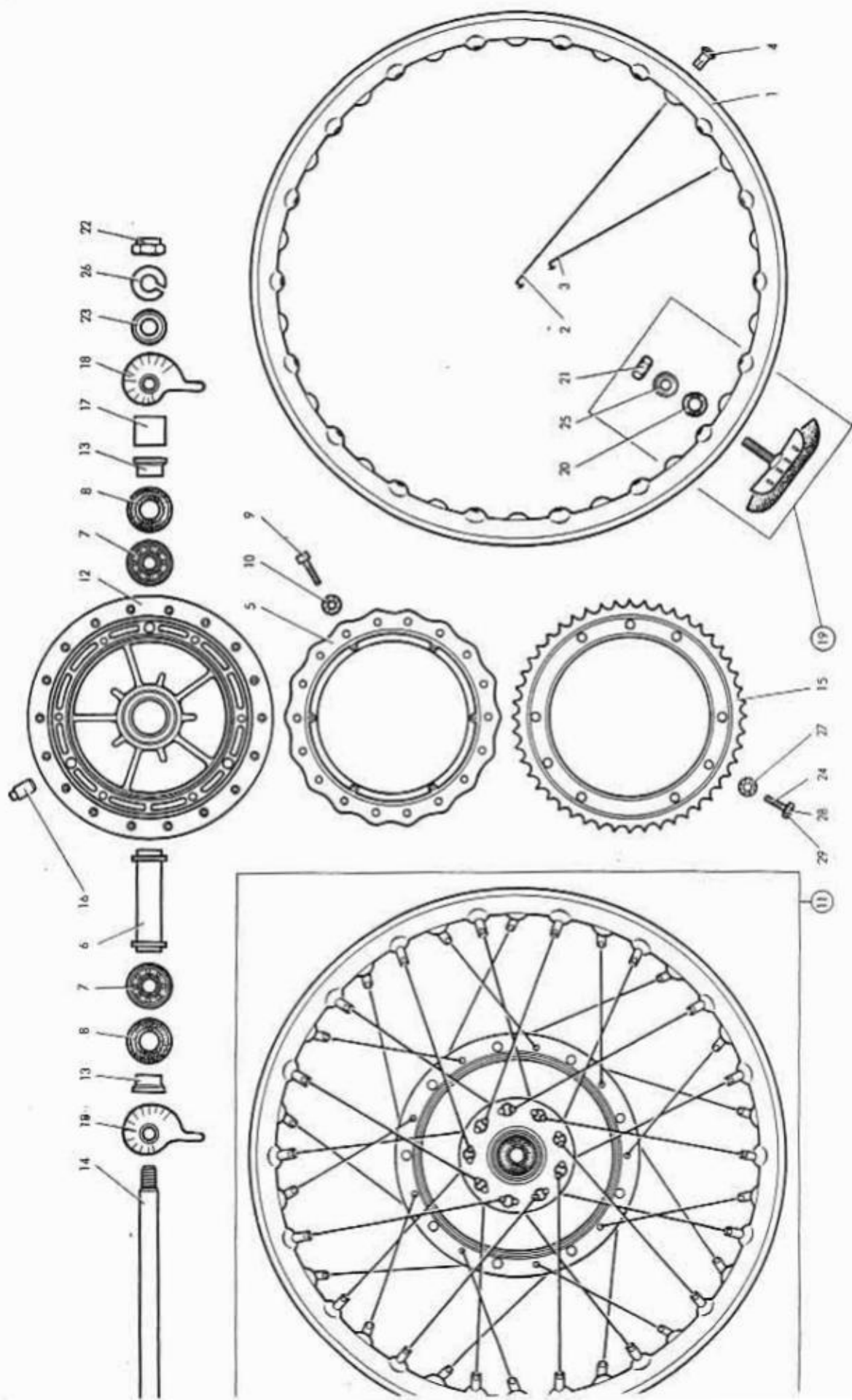
RUEDA TRASERA
