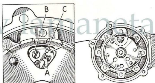
Fig. Z4. Adjusting the Contact Breaker Points (Lucas).
