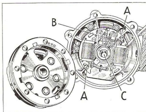
Fig. Z5. Generator (Lucas).
