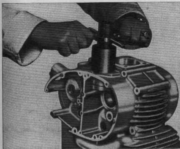
3 - Estrattore per bussola portacuscinetti 88713.0252
