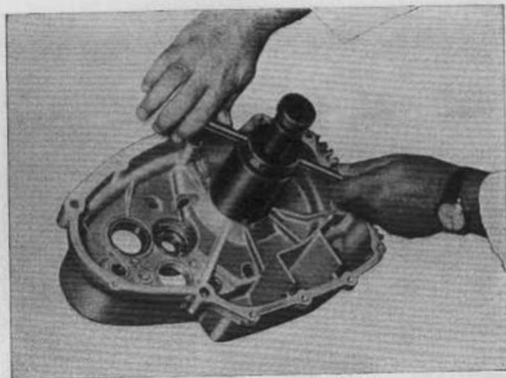
24 - Estrattore per cuscinetti 83713.0269
