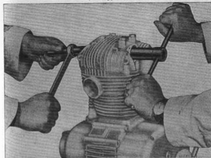
15 - Chiave fissa-albero distribuzione per bloccare ingranaggio conico Z=28 88713-0253
