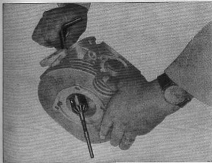
22 - Frese per sedi valvole (vedi leggenda)
