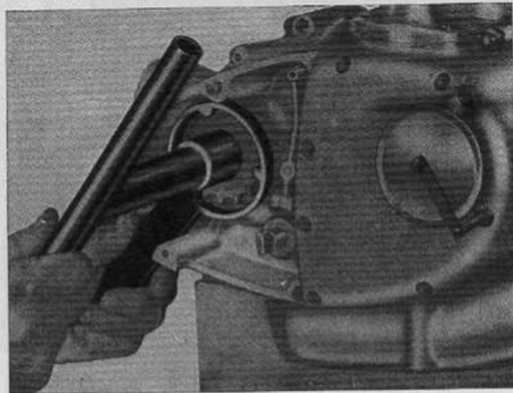
6 - Chiave fissa-pignone Z=12 per bloccaggio dado 88713.0462
