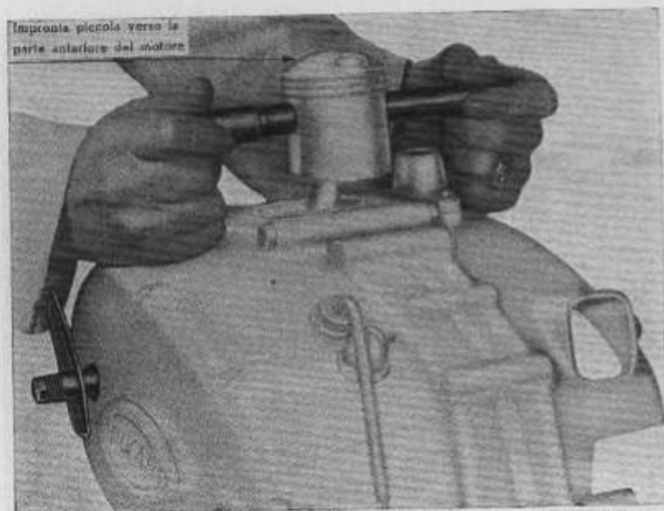
16-17 - Spina per montaggio e smontaggio spinotto pistone 88713.0450/0431
