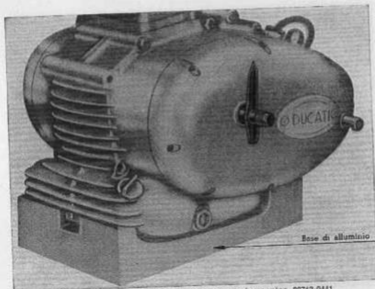
10 - Indice controllo anticipo per luce stroboscopica 88713-0441
