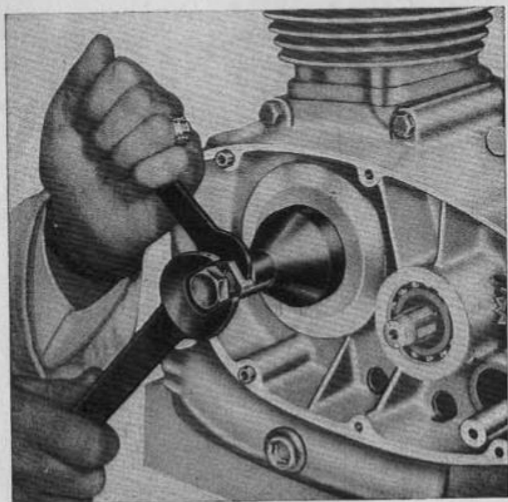
1 - Estrattore per volano 88713.0411
