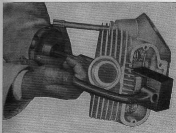
21 - Attrezzo per montaggio e smontaggio valvole 88713.0267
