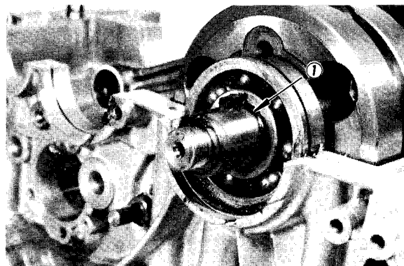
1. Kurbelwellendichtung
