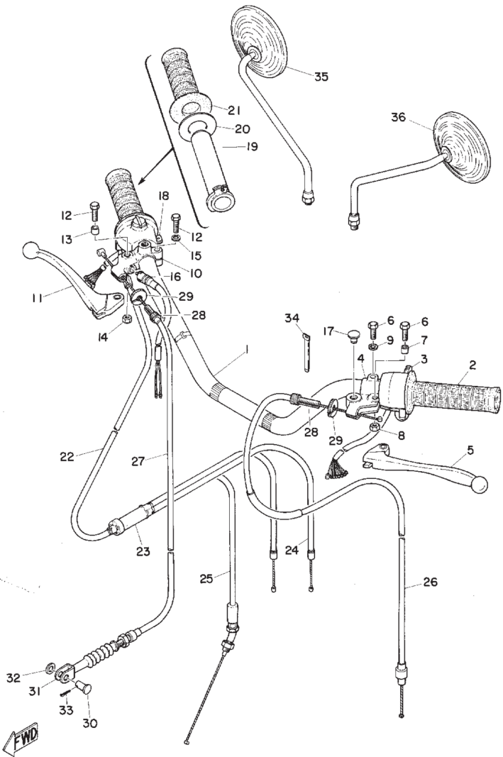
Fig. 24 HANDLE · WIRE
