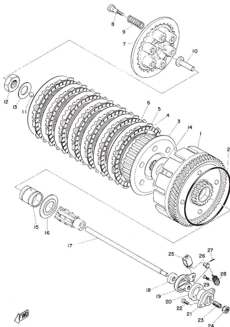
Fig. 5 CLUTCH
