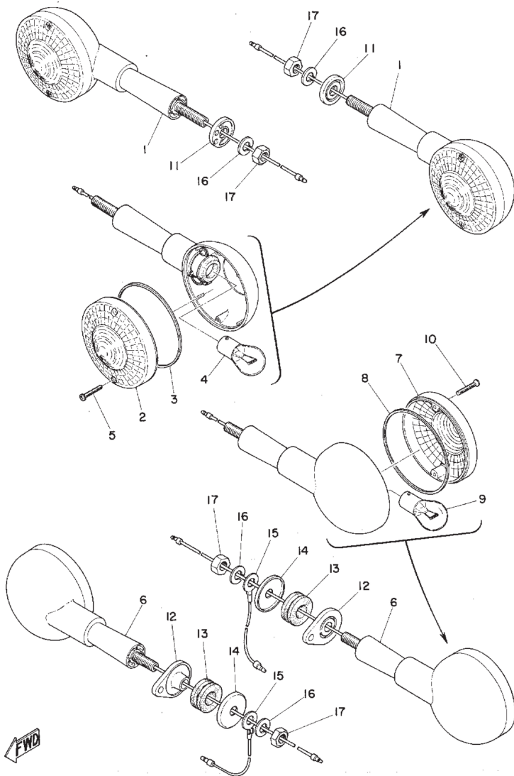
Fig. 36 FLASHER LAMP
